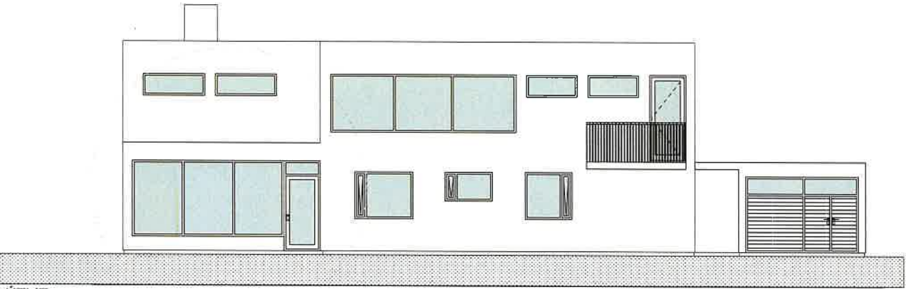
ÚTLIT SUÐUR
