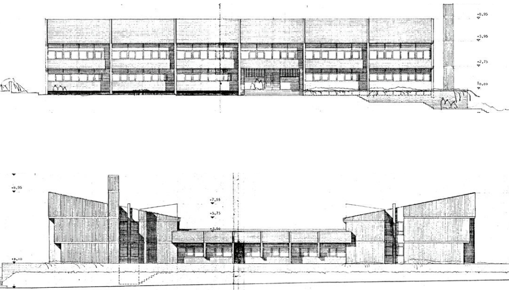
Mynd 162: Ásýndir. Aðaluppdráttur Þinghólsskóla, 1971.
