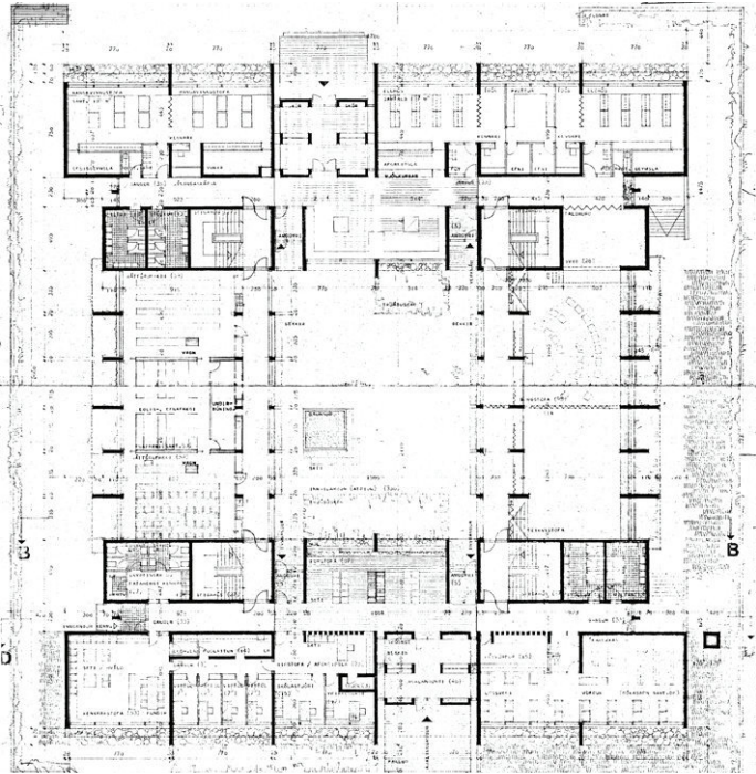
Mynd 165: Grunnmynd jarðhæðar. Aðaluppdráttur Þinghólsskóla, 1971.
