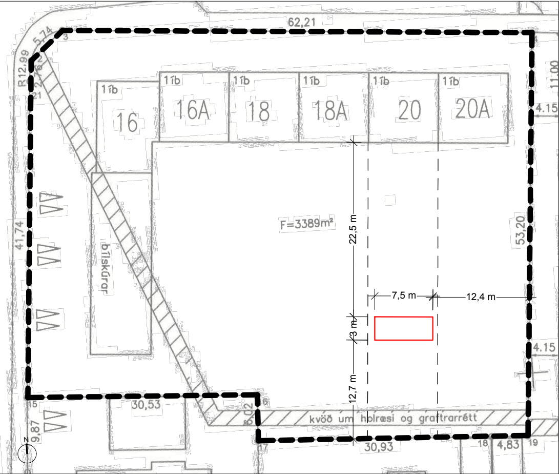
Tillaga að breytingu: afstöðumynd mkv 1:500
