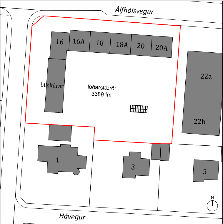
Tillaga að breytingu: Álfrólsvogur 20, mkv. 1:1000
