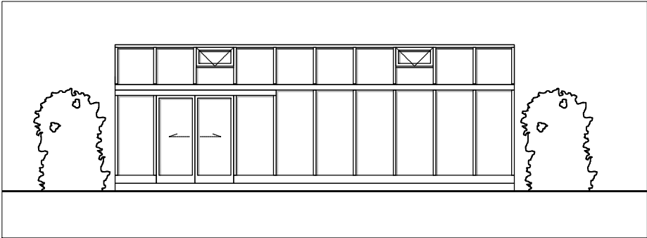
Tillaga að breytingu: norður- og suðurhlíð mkv 1:100
