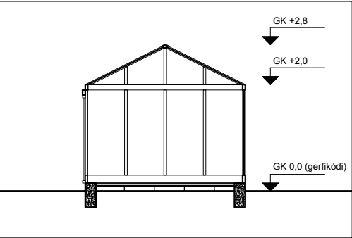
Tillaga að breytingu: snið mkv 1:100
