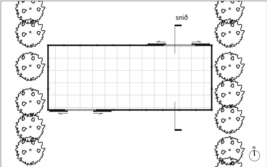
Tillaga að breytingu: grunnmynd mkv 1:100
