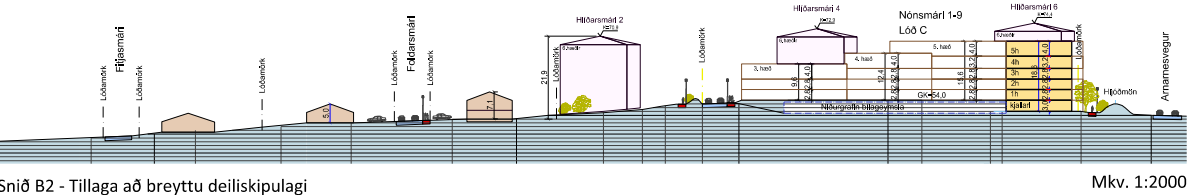
Snið B2 - Tillaga að breyttu deiliskipulagi Mkv. 1:2000
