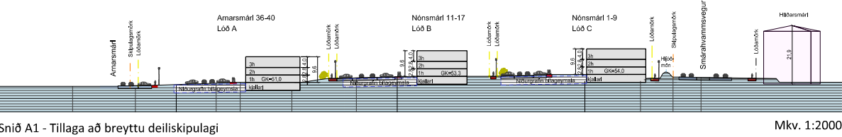
Snið A1 - Tillaga að breyttu deiliskipulagi Mkv. 1:2000
