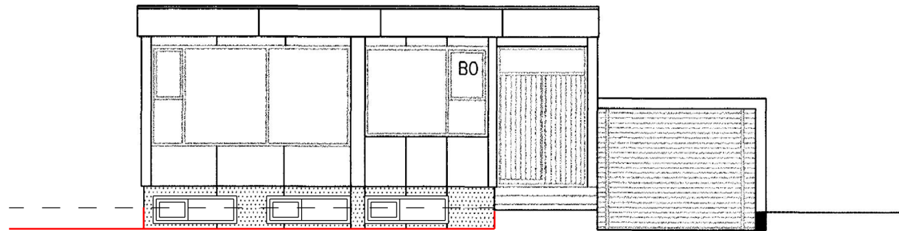
NORDUR ÚTLIT EFTIR
