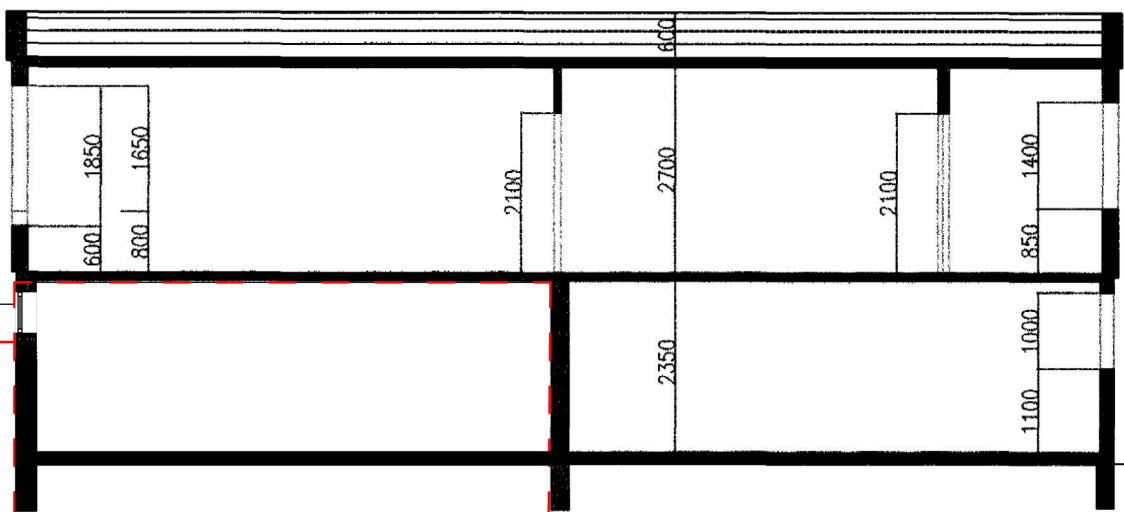
SKURDUR B-B SNID EFTIR
