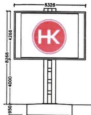
AUGLÝSINGAMASTUR ÁSÝND MKV. 1:100
