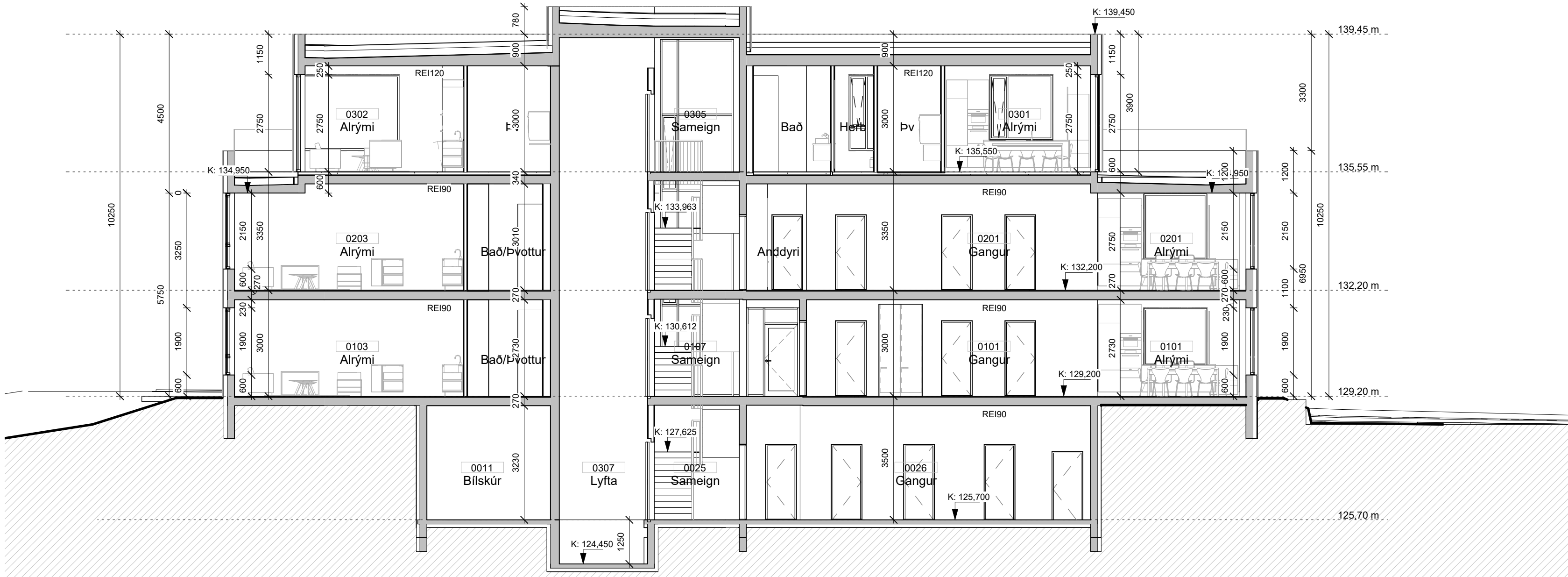
Snið 1 1 : 100
