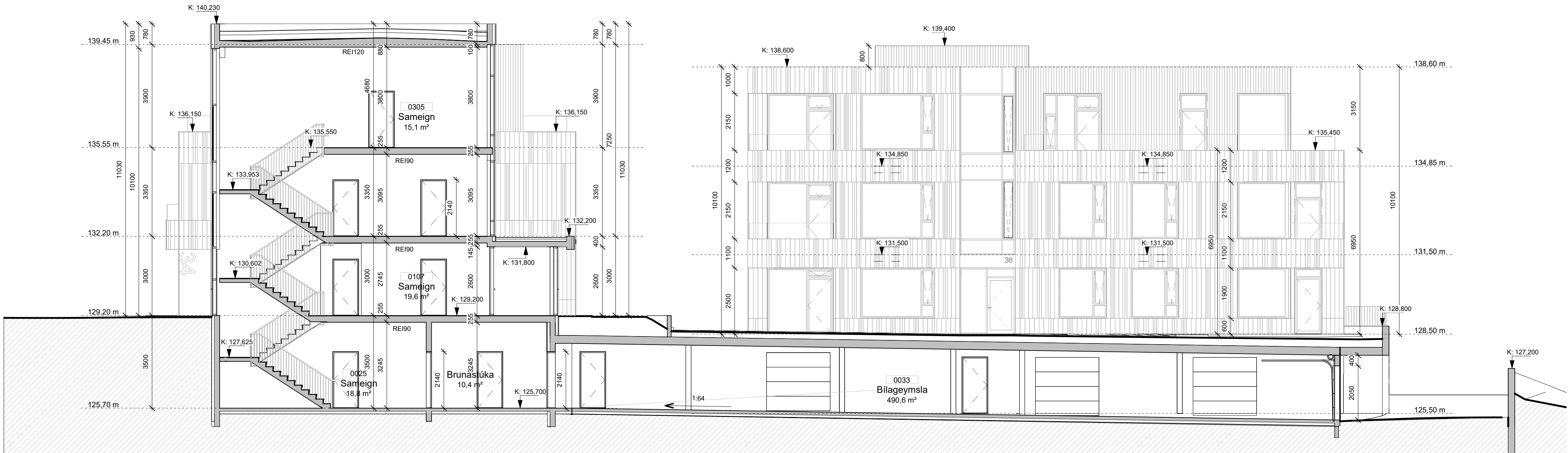
Snið A 1 : 100
