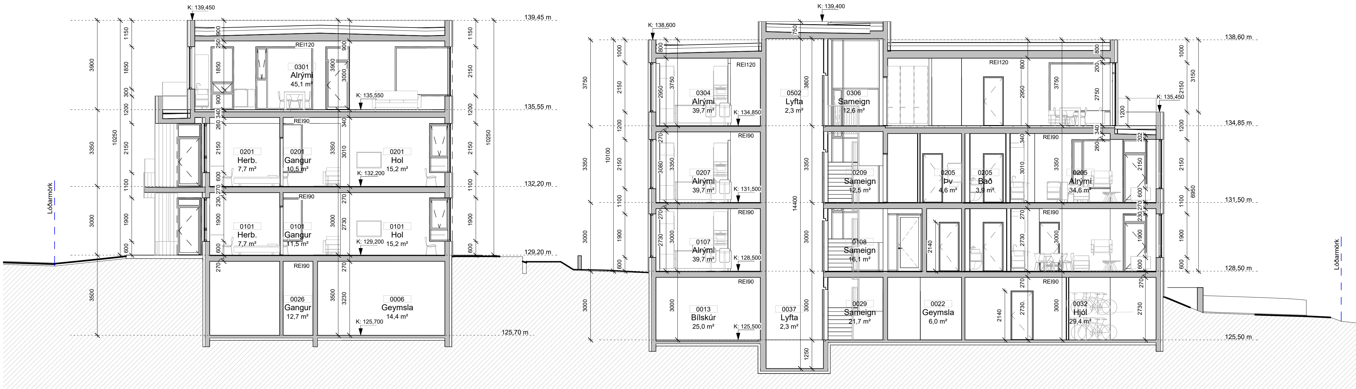
Sníð B 1 : 100
