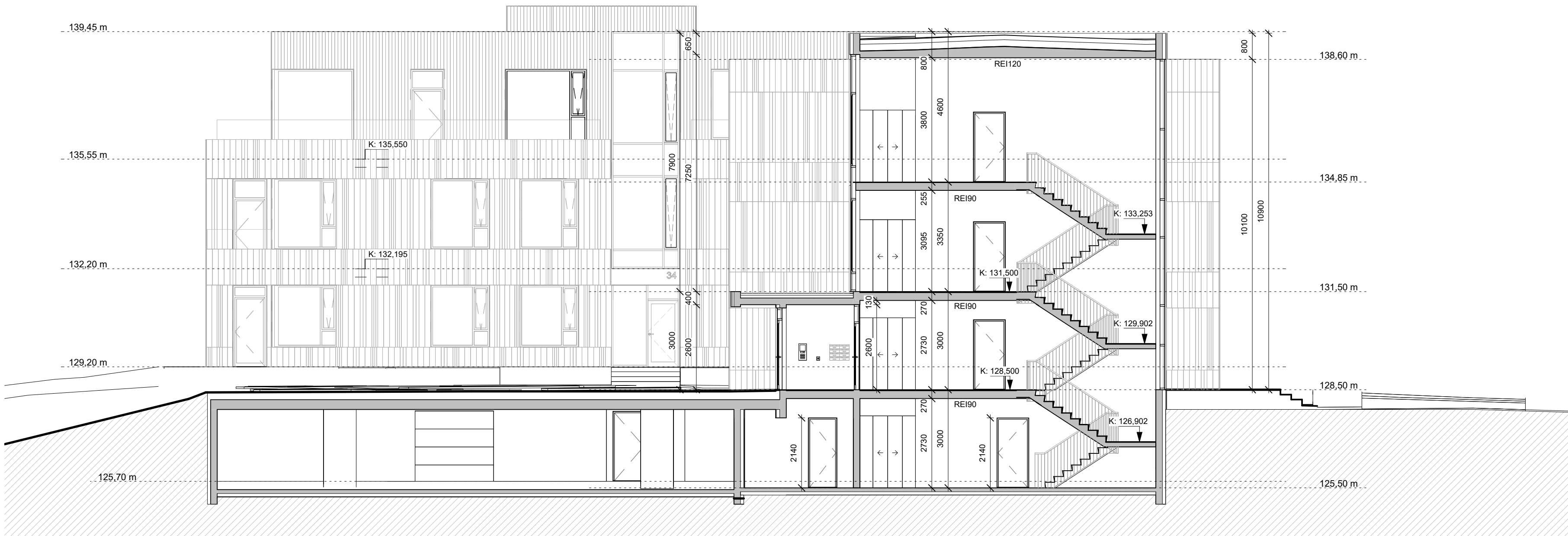
Sníð 2 1 : 100
