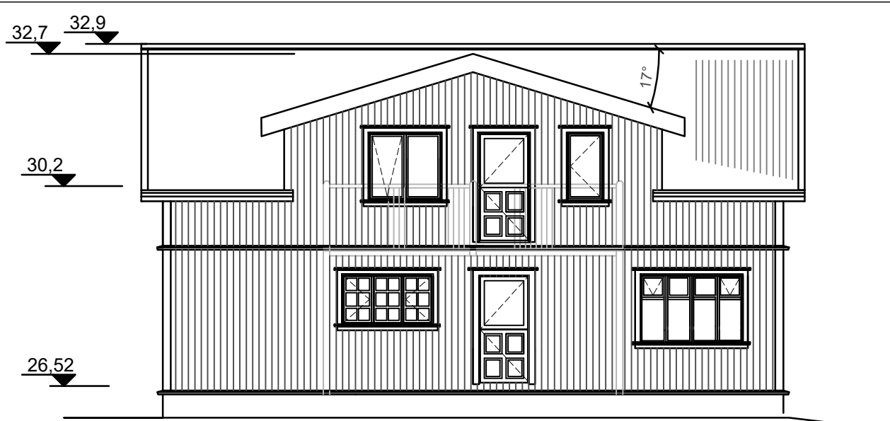
Útlit Suður
