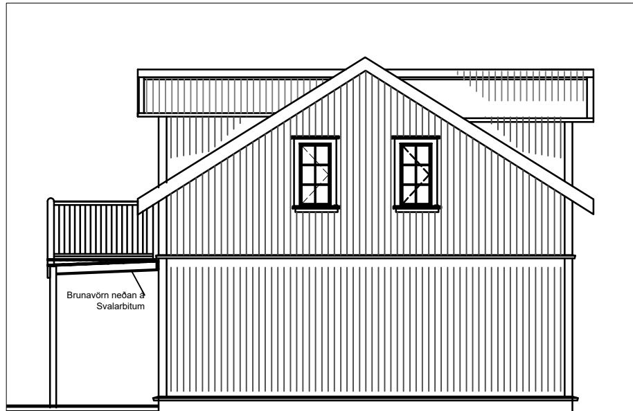
Útlit Austur
