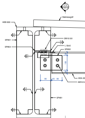
ST7a Sníð 1:5
