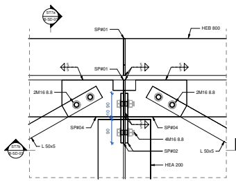
ST7 Særmýnd 1:5
