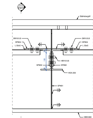
ST7a Sníð 1:5
