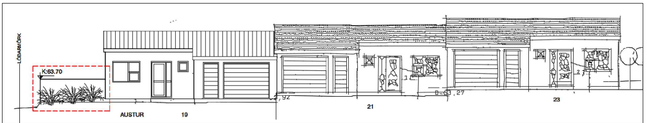
Skýringarmynd: Tillaga - Útlit til austurs. mkv. 1:500
