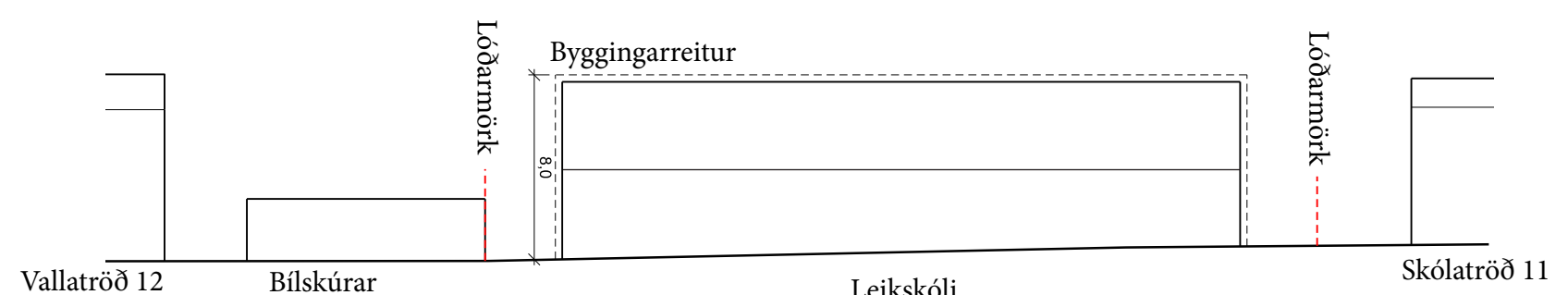
Sneiðing b-b
