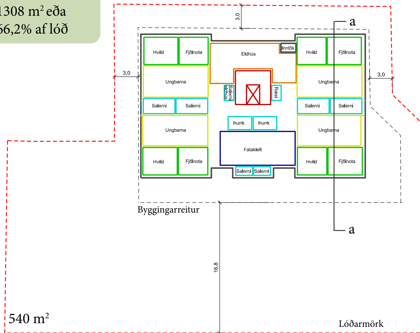
1. Hæð
