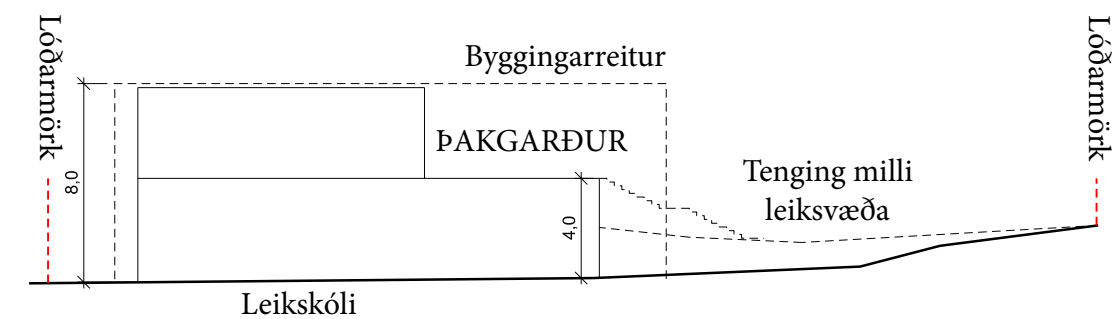
Sneiðing a-a
