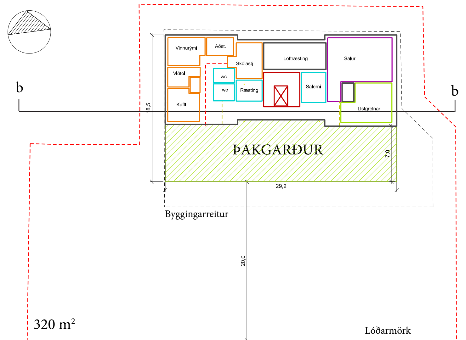
2. Hæð
