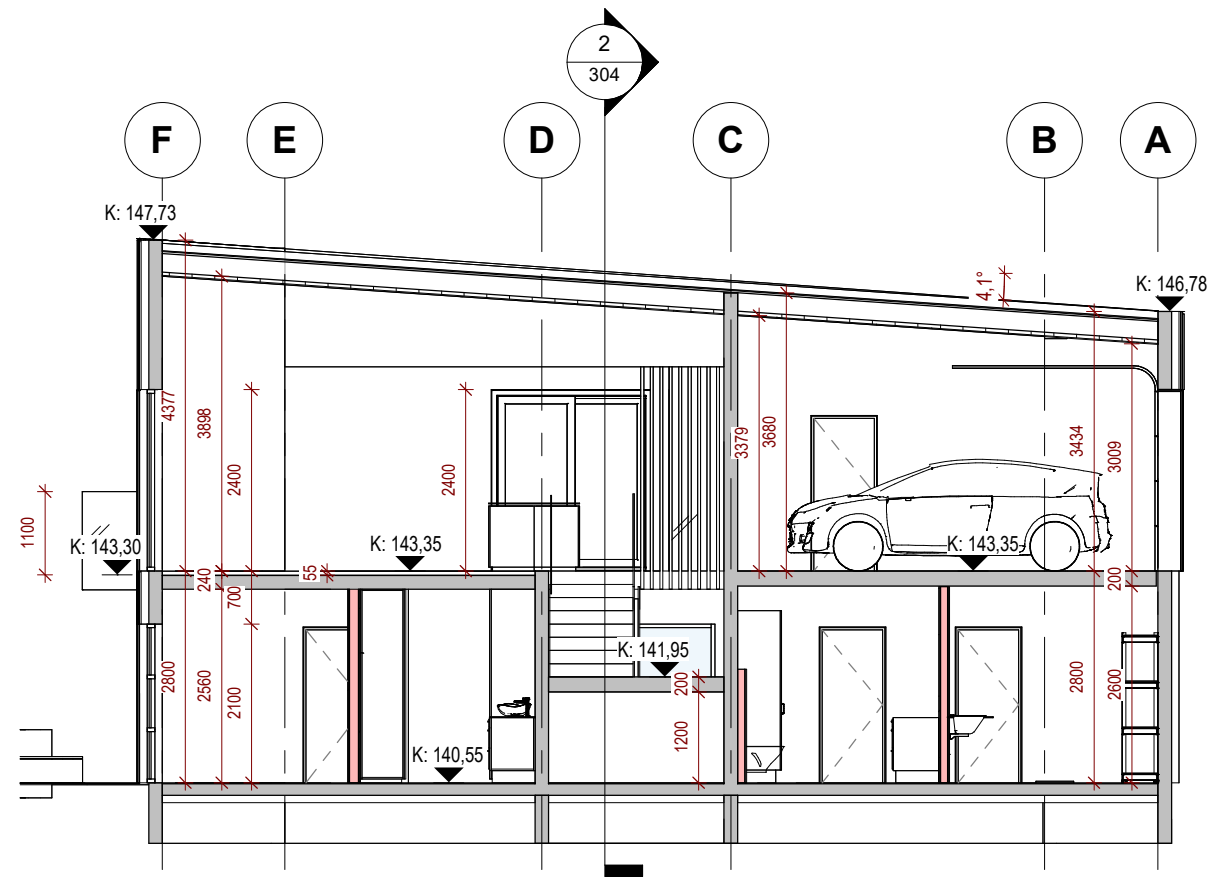
1 SNID A-A 1 : 100
