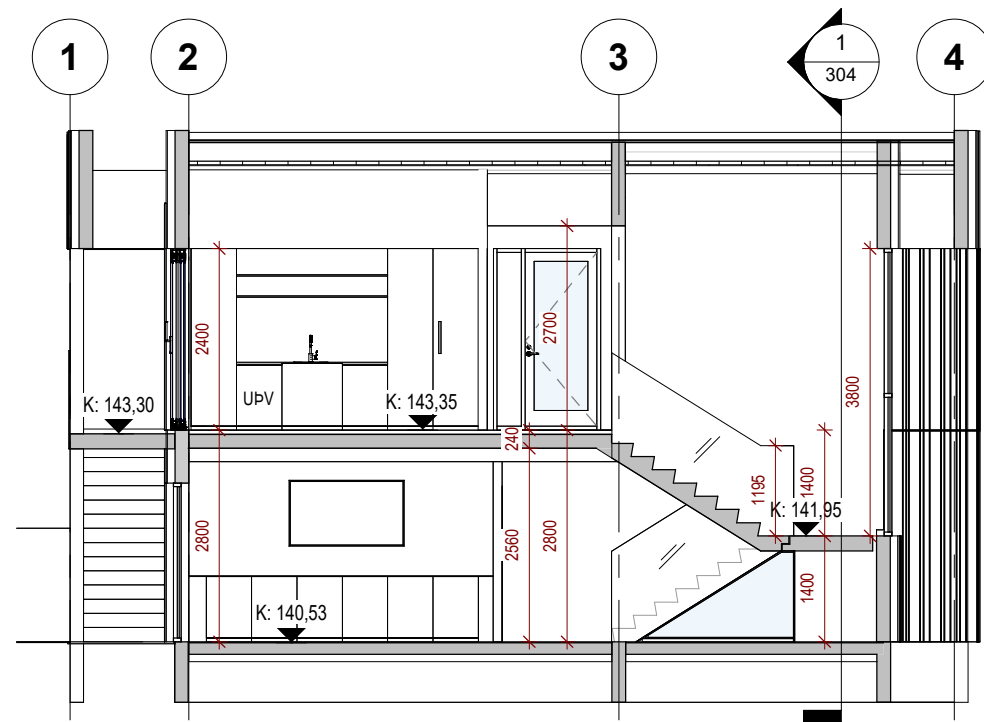
2 SNID B-B 1 : 100
