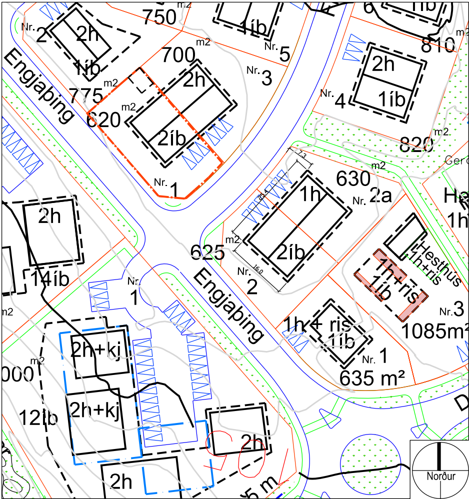
Tillaga að breyttu deiliskipulagi: Frostþing 1. í mkv. 1:1000
