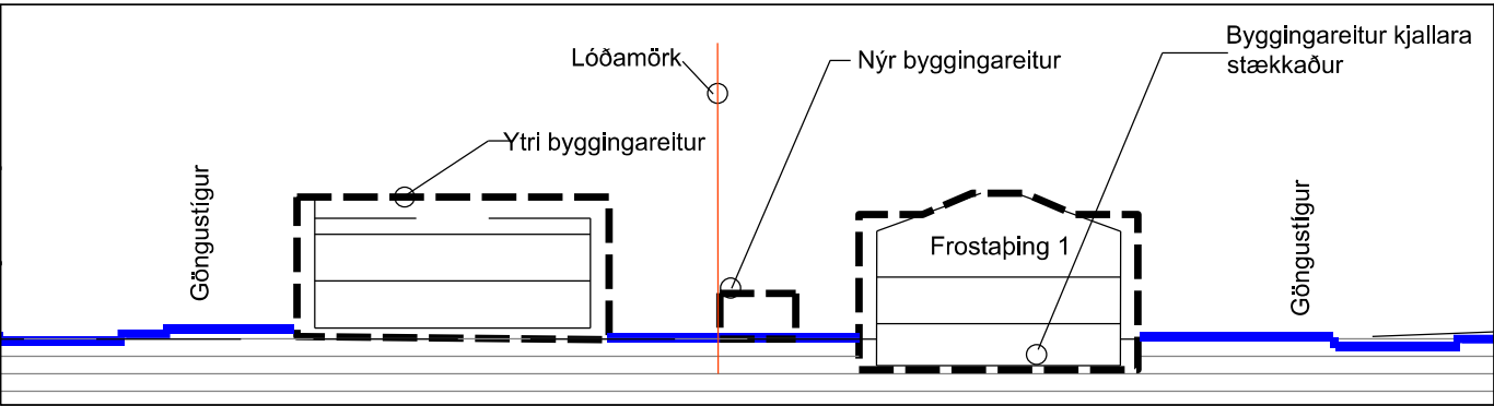
Tillaga að breyttu deiliskipulagi: Sneiðmynd A-A í mkv. 1:500
