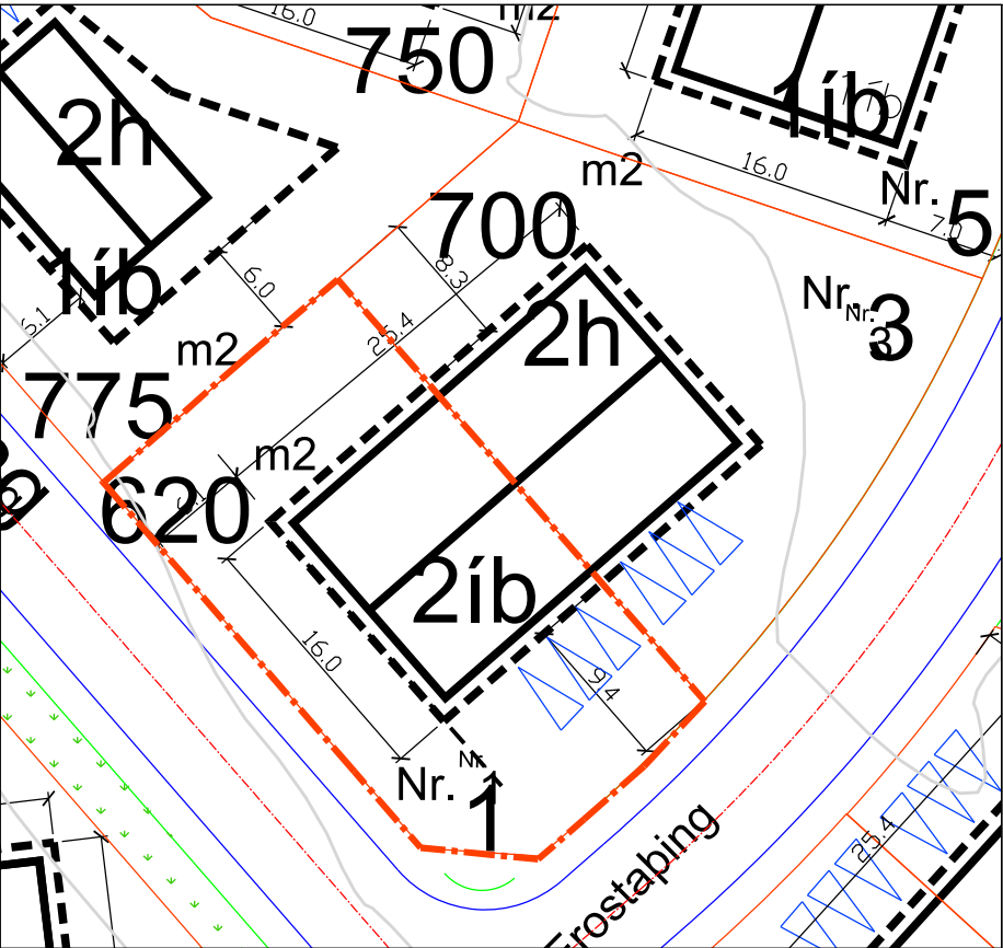
Skýringarmynd: Afstöðumynd Frostþings 1, í mkv. 1:500
