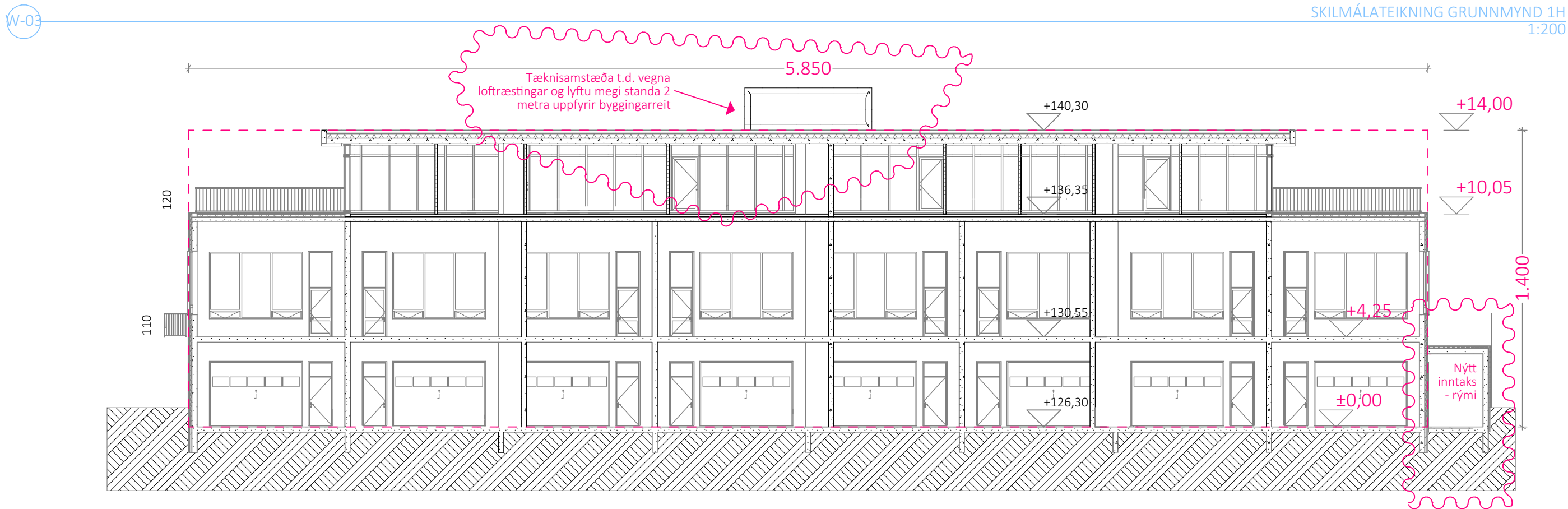
SKILMÁLATEIKNING SNÍÐ 1 1:200
