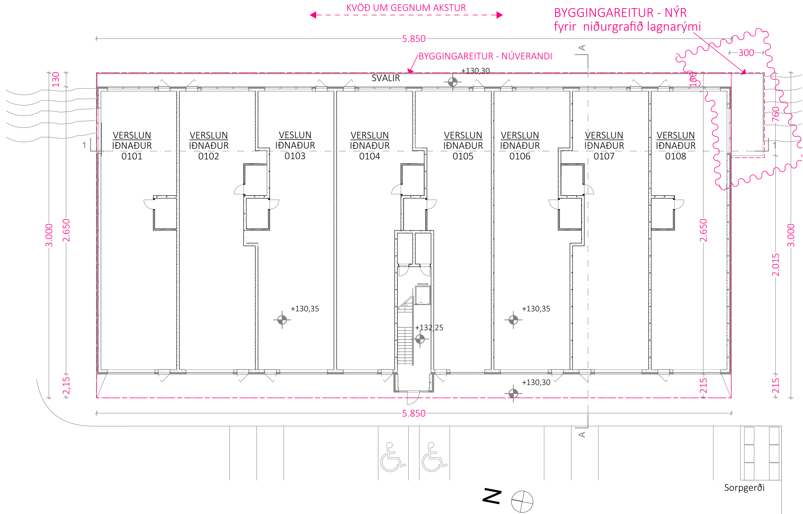
SKILMÁLATEIKNING GRUNNMYND 1H 1:200
