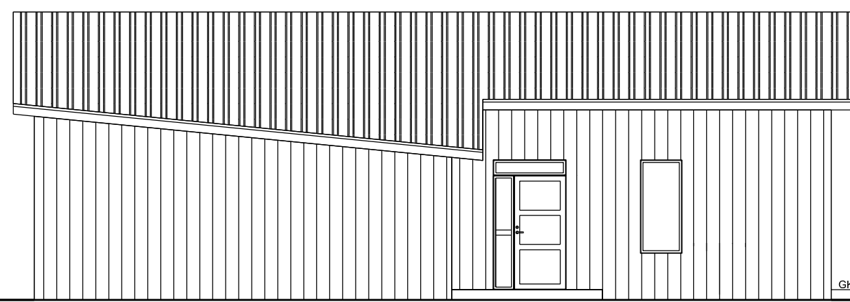
ÚTLIT Í NORÐUR
