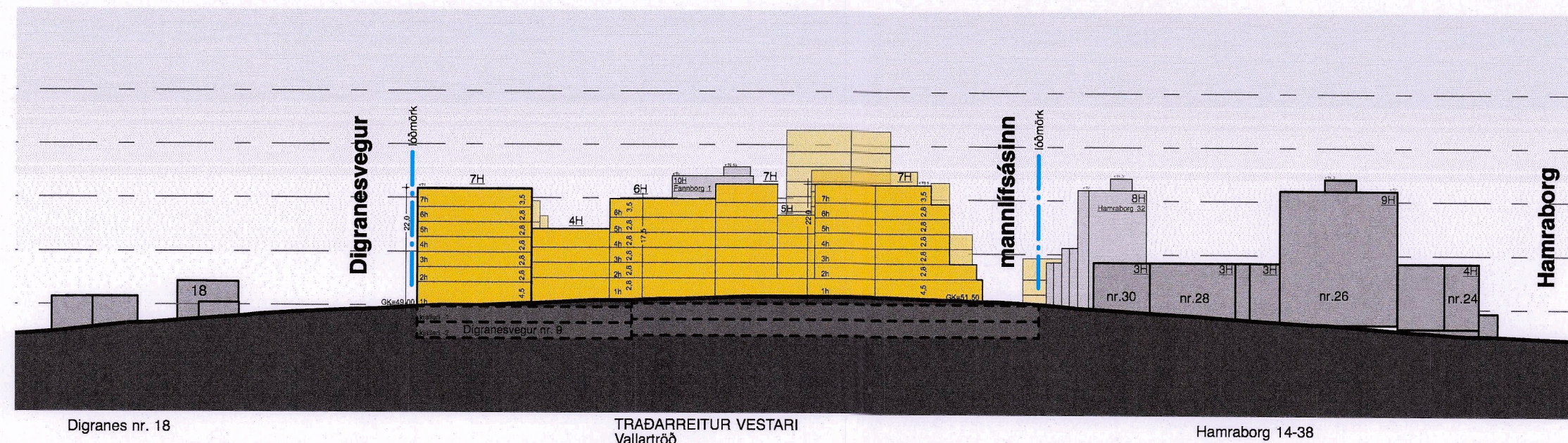
SKILMÁLASNEIÐING A-A VALLARTRÖÐ
