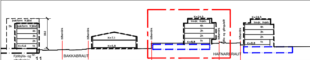
Hluti úr gildandi deiliskipulagi: Skýringarmynd Sneiðing Þ-1 Mk. 1:1000
