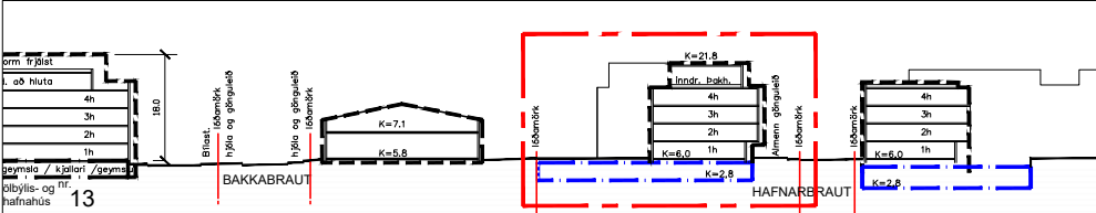
Tillaga að breyttu deiliskipulagi: Skýringarmynd Sneiðing Þ-2 Mk. 1:1000
