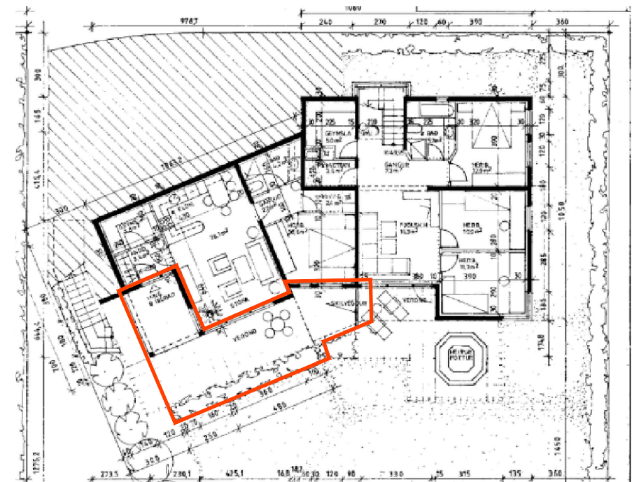
Núv. grunnmynd kjallara mkv.1:250 og mörk stækkunar kjallara.
