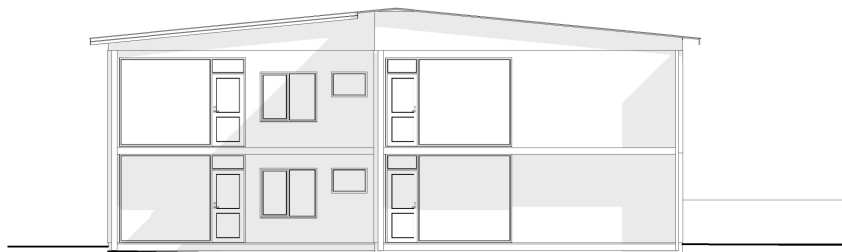
③ Suður Mkv. 1 : 100
