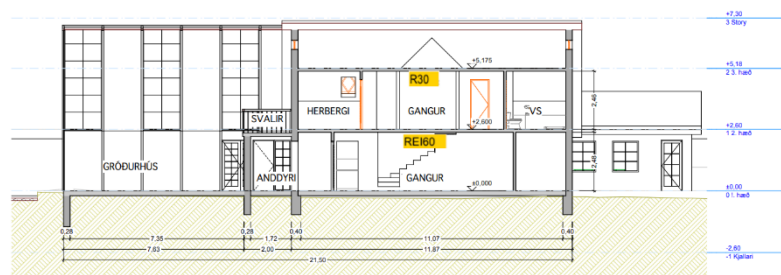
SKURÐUR C-C
