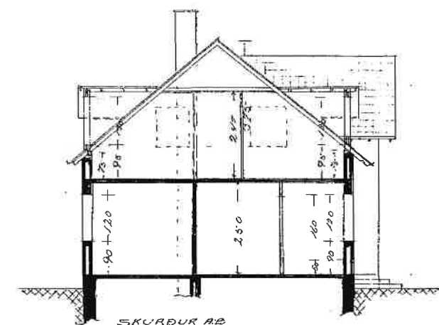
SKURÐUR A2
