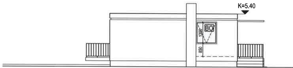
ÚTLIT, NORÐAUSTURHLIÐ, 1:100
