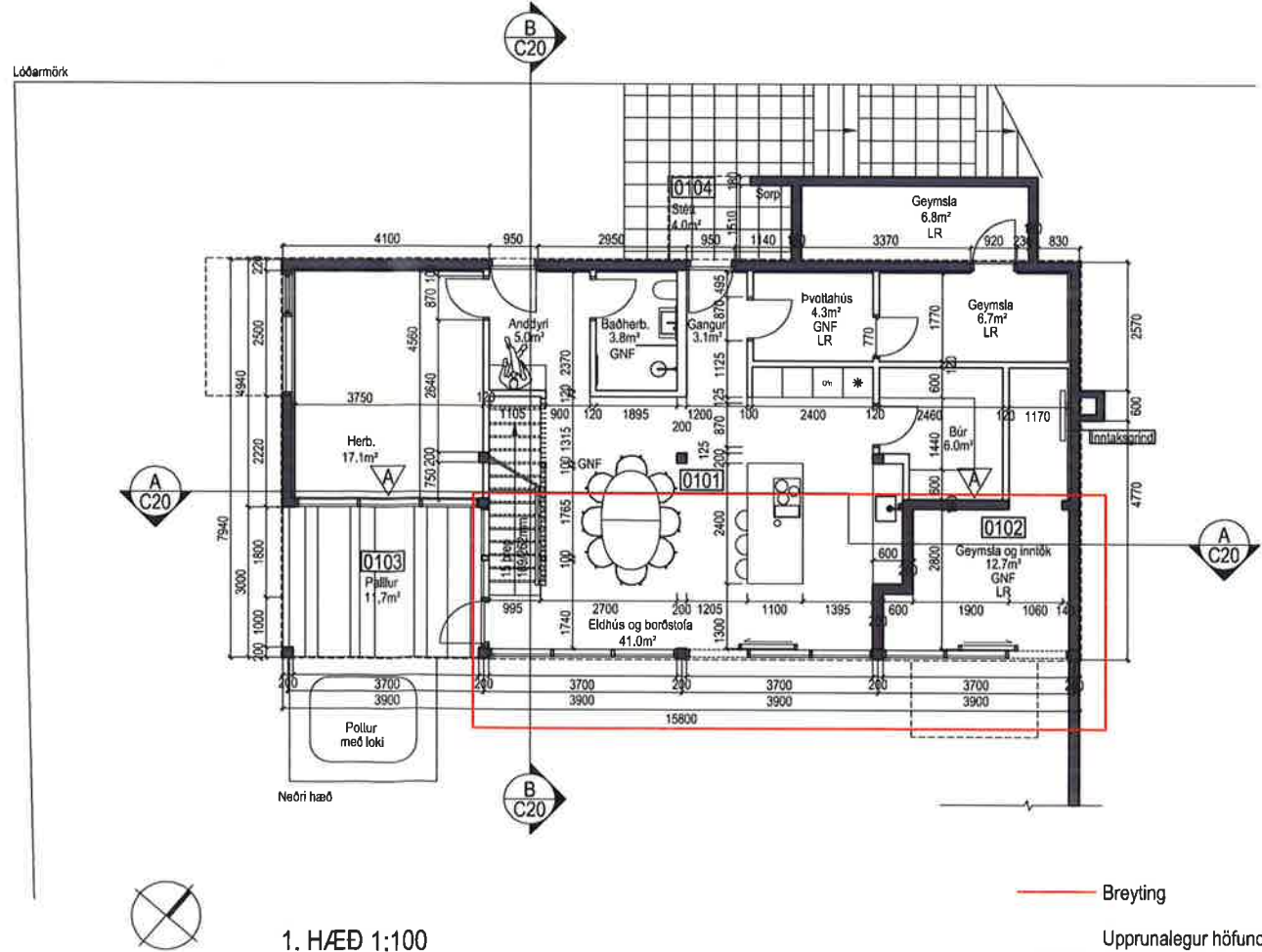
1. HÆÐ 1:100
