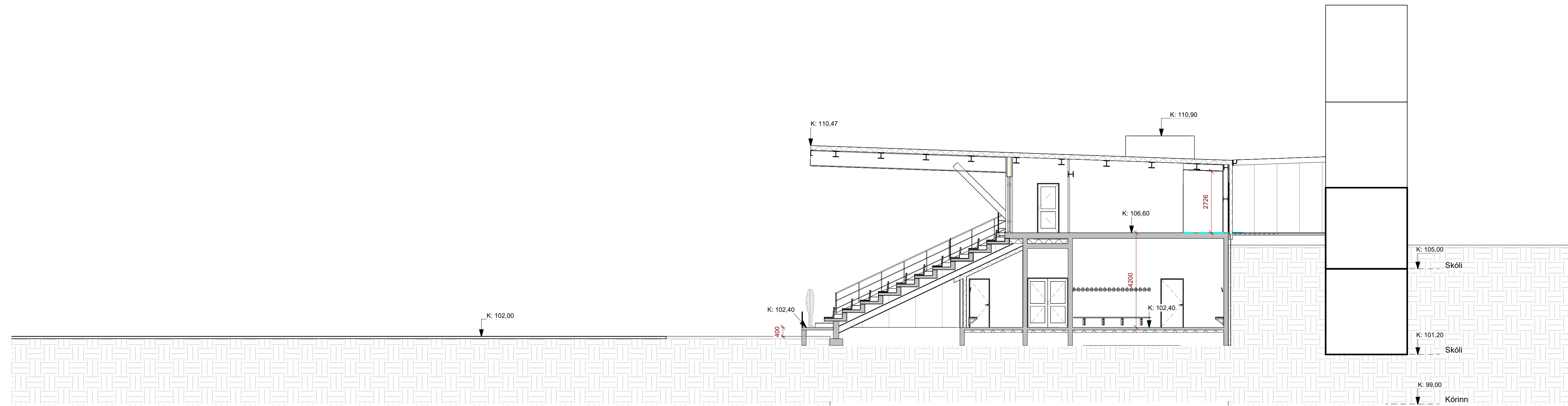
2 Snið B-B 1 : 100
