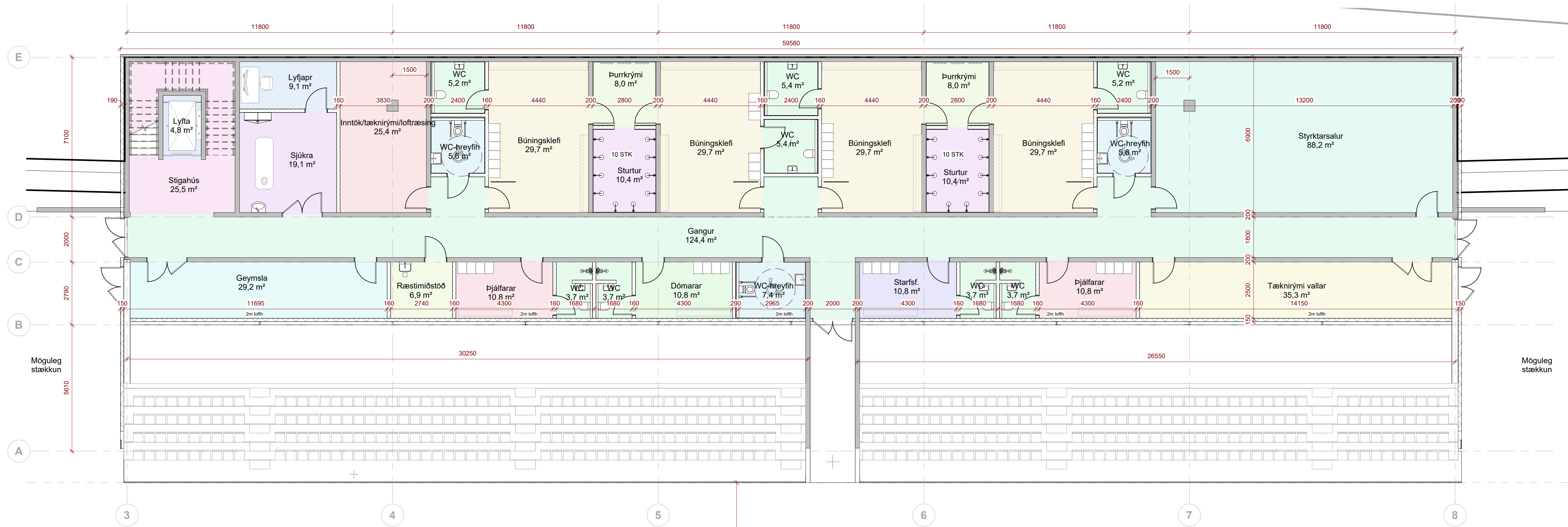
1. hæð - lituð 1: 100
