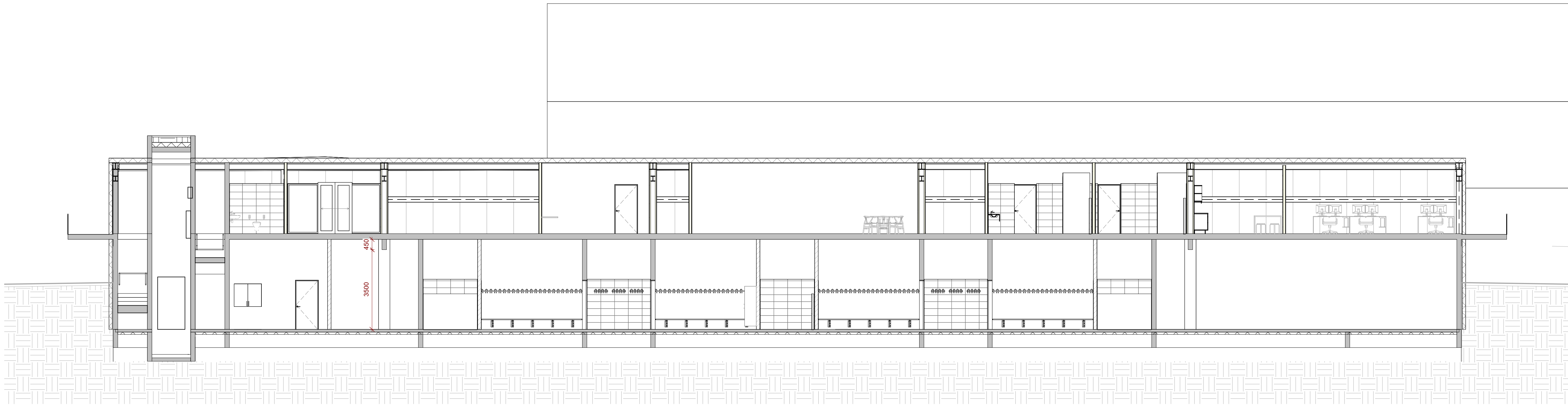
1 Snið C-C 1 : 100
