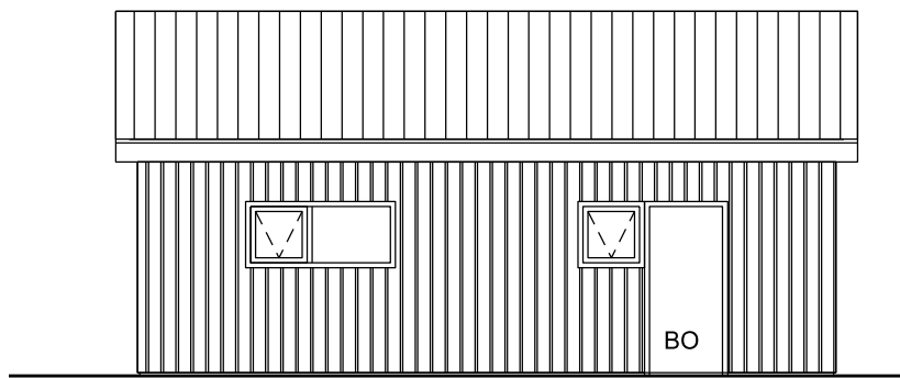
ÚTLIT Í AUSTUR
