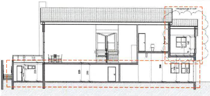
Snið
