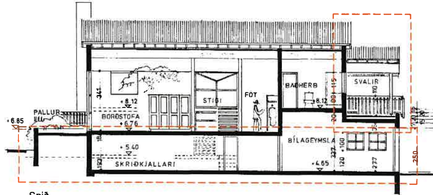
Snið
