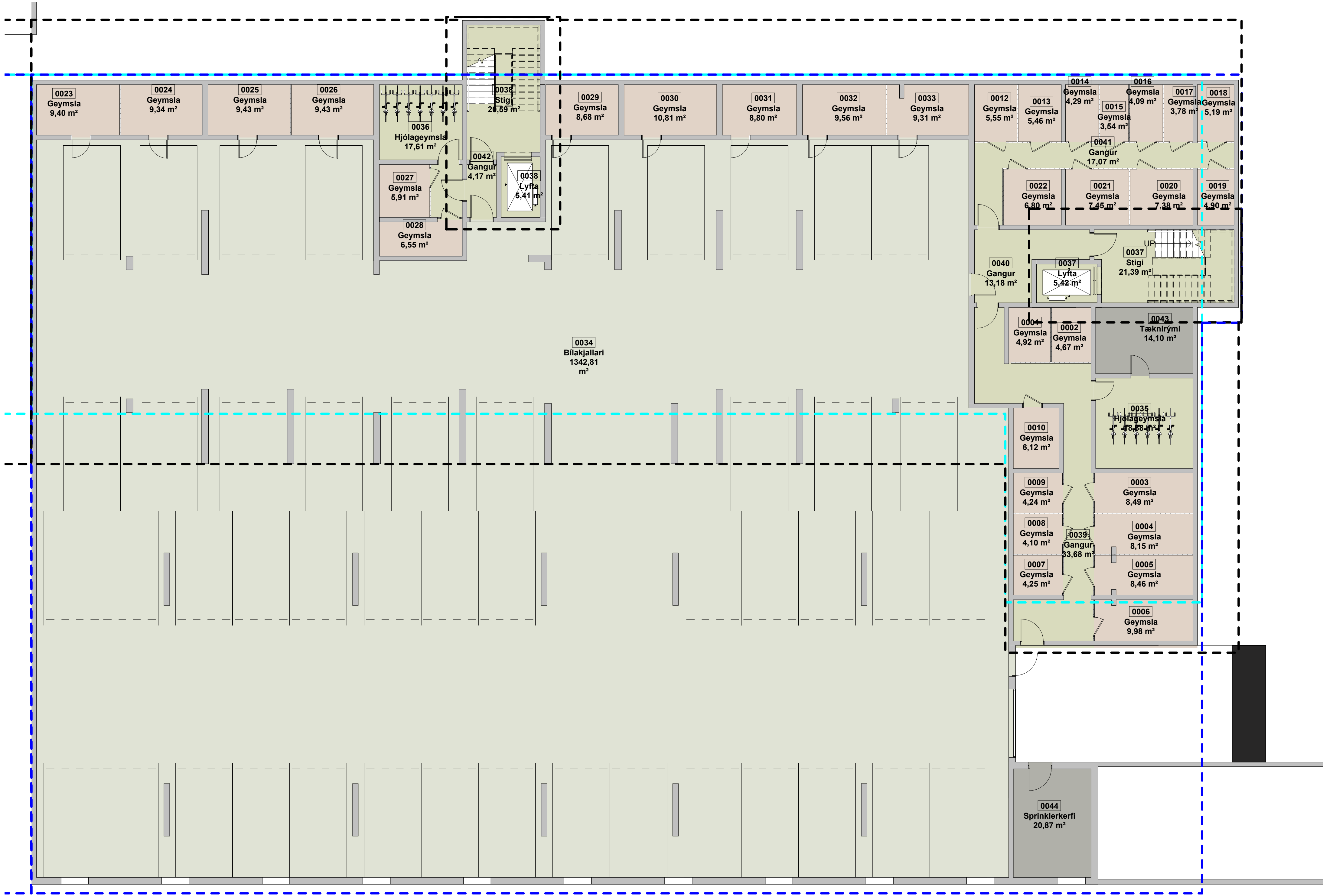
FT-Kjallari, brúttó 1 : 100
