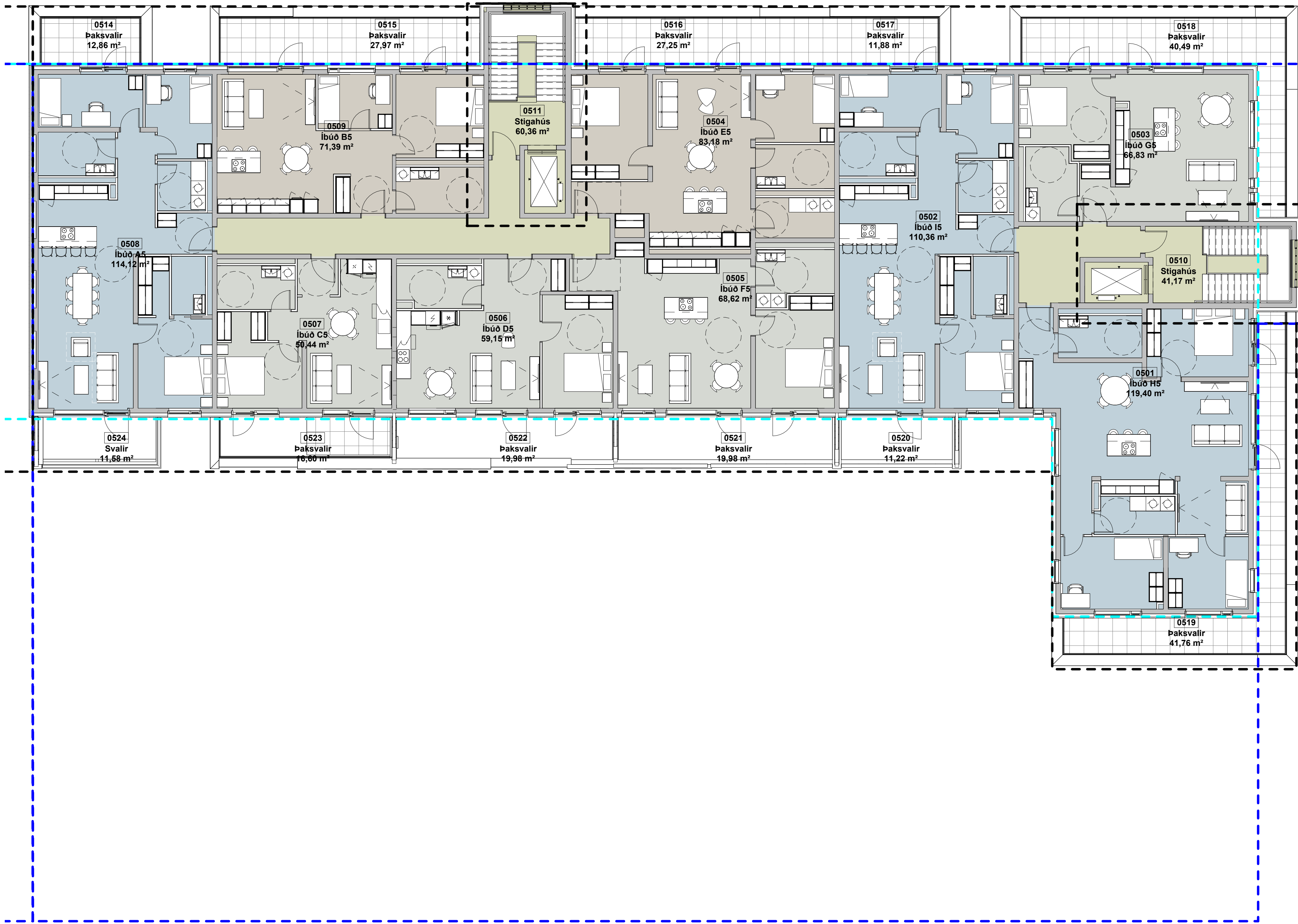
FT-5. hæð, brúttó 1 : 100
