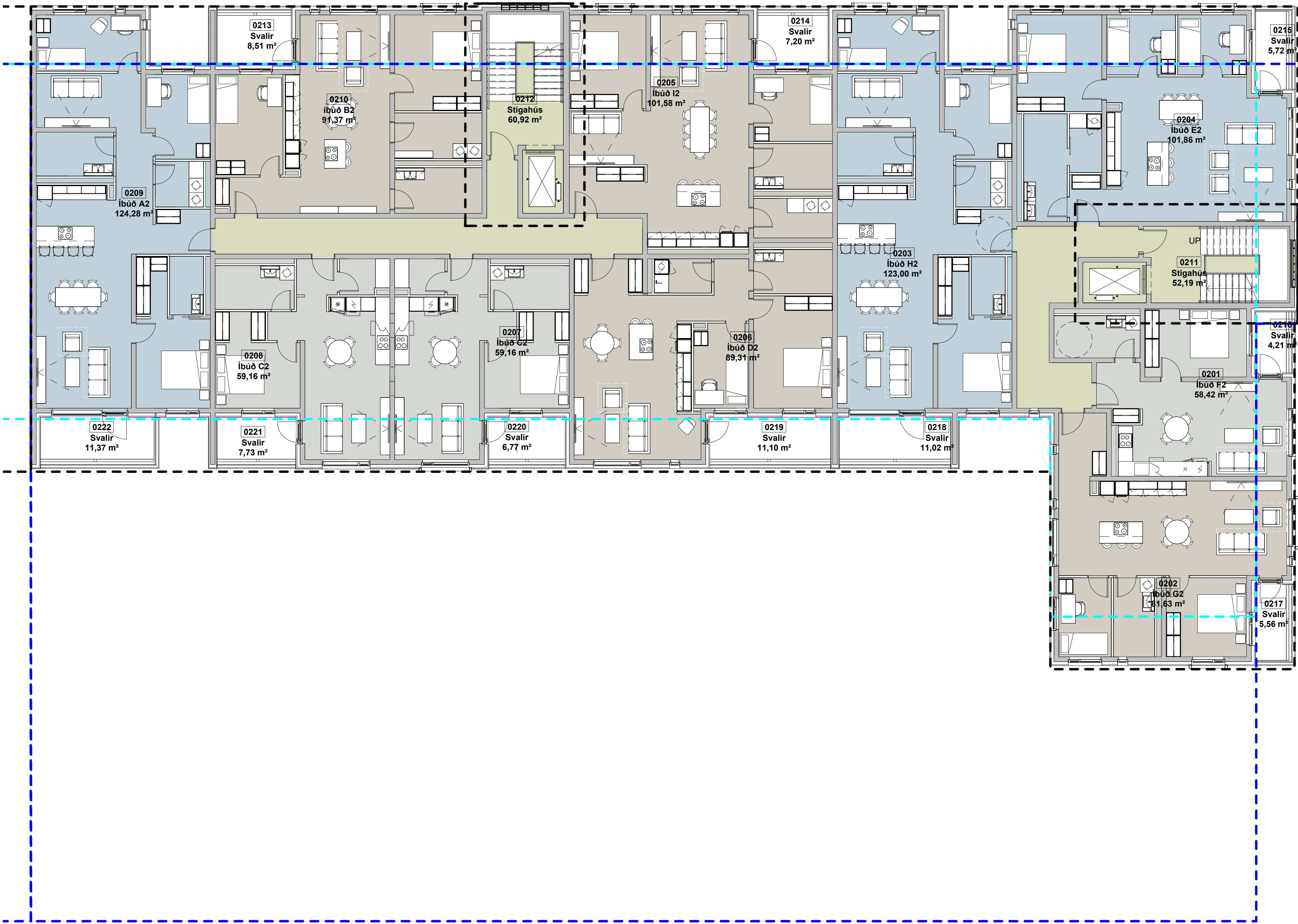
FT-2. hæð, brúttó 1 : 100
