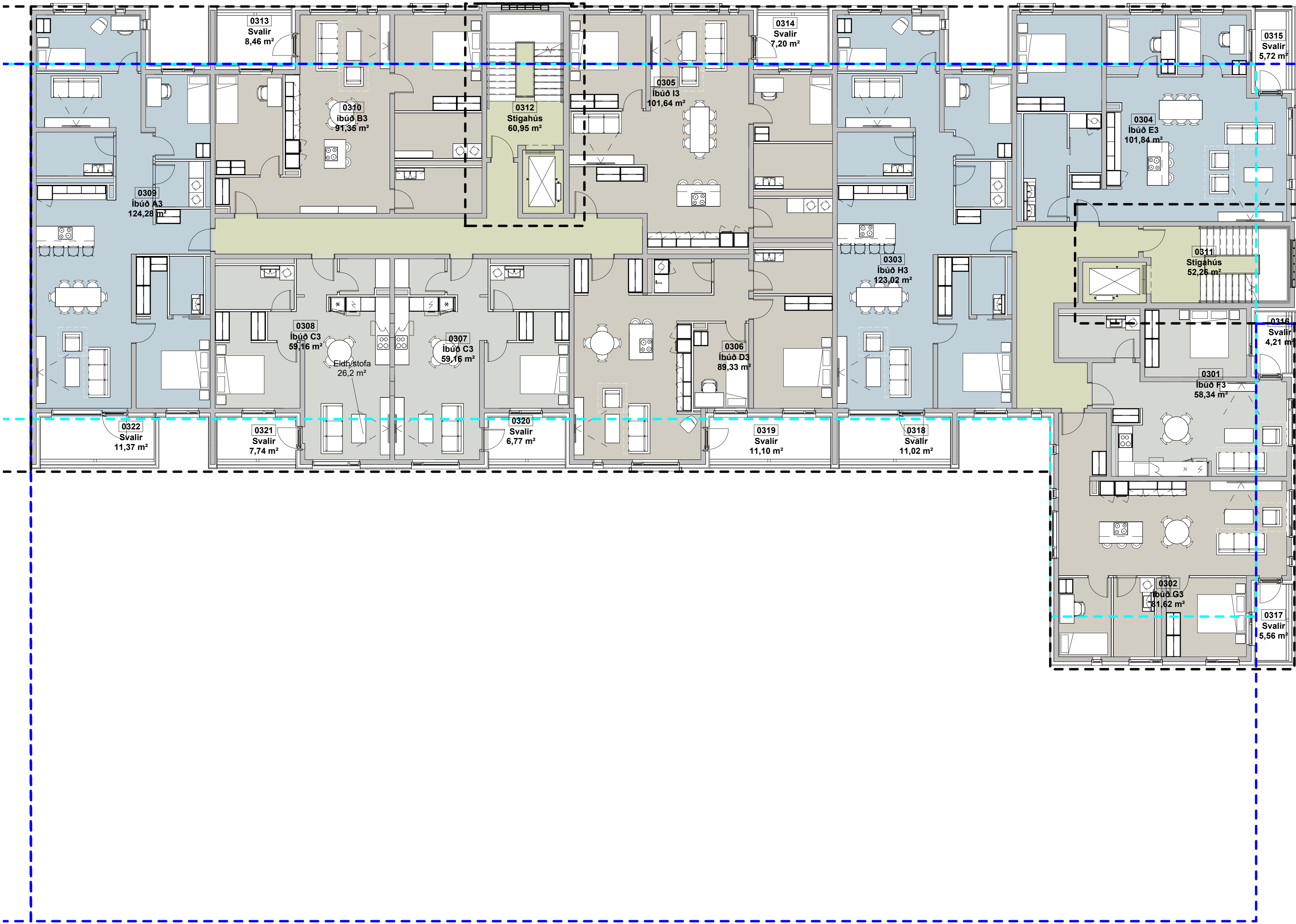
FT-3. hæð, brúttó 1 : 100
