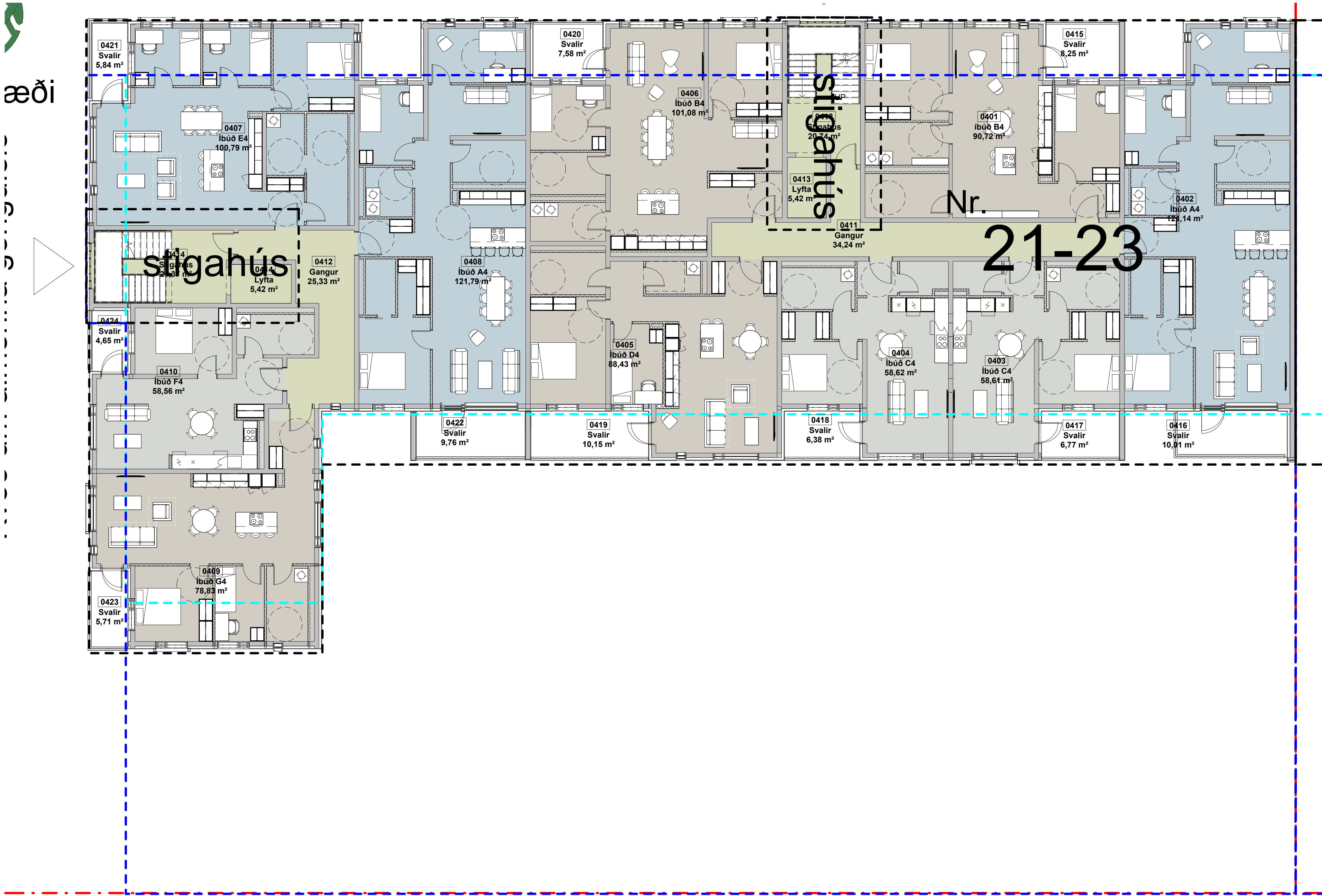
FT-4. hæð, brúttó 1 : 100
