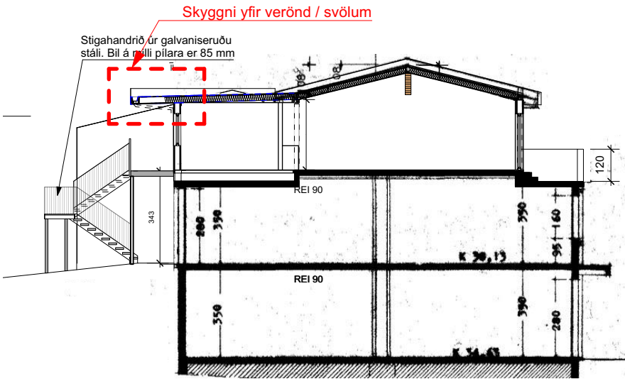
SNEIÐING EFTIR BREYTINGU
