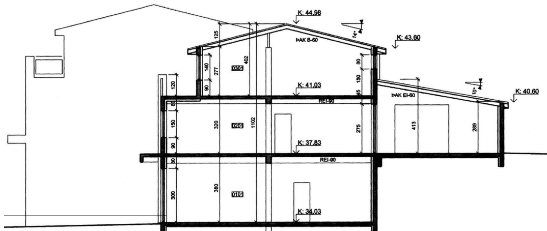
VESTURHLIÐ FYRIR BREYTINGU
