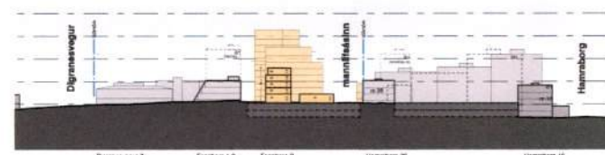
SKILMÁLASNEIÐING F-F
