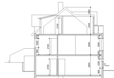
Skurðmynd
