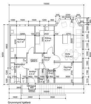
Grunnmynd kjallara
