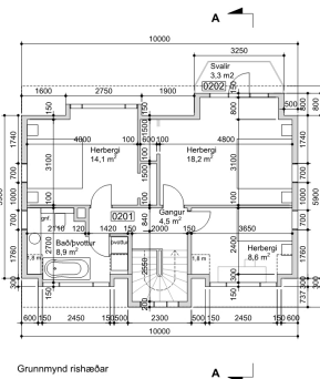
Grunnmynd rishæð
