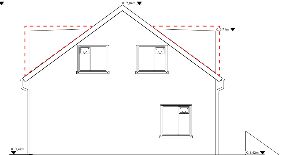
AUSTURHLID 1:100
