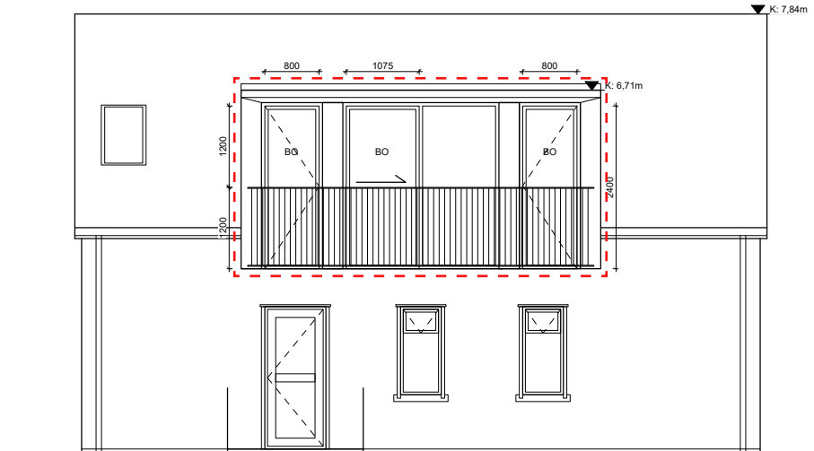
NÖRÐURHLID 1:100
