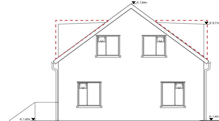
VESTURHLID 1:100
