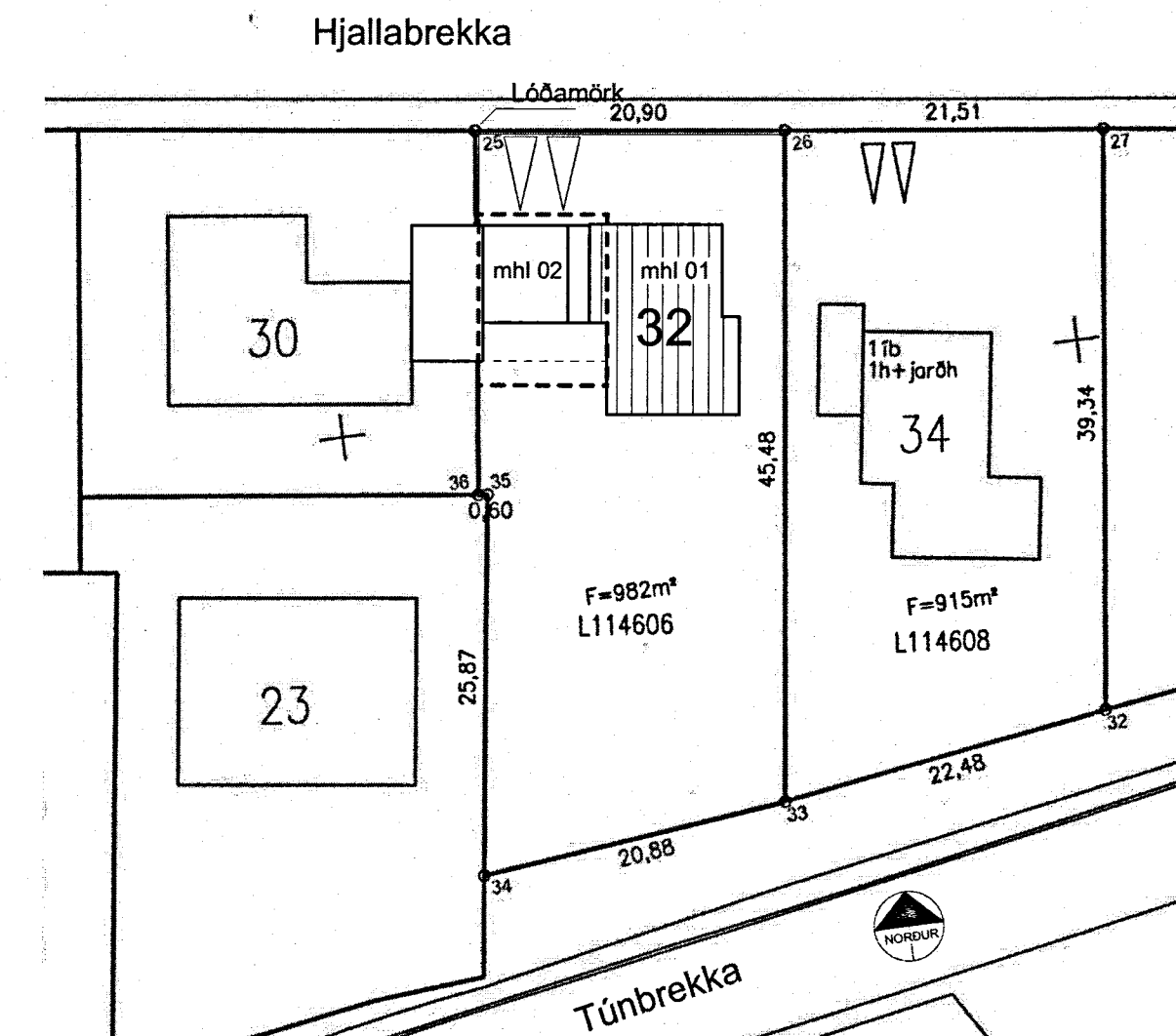
Afstöðumynd 1:500
