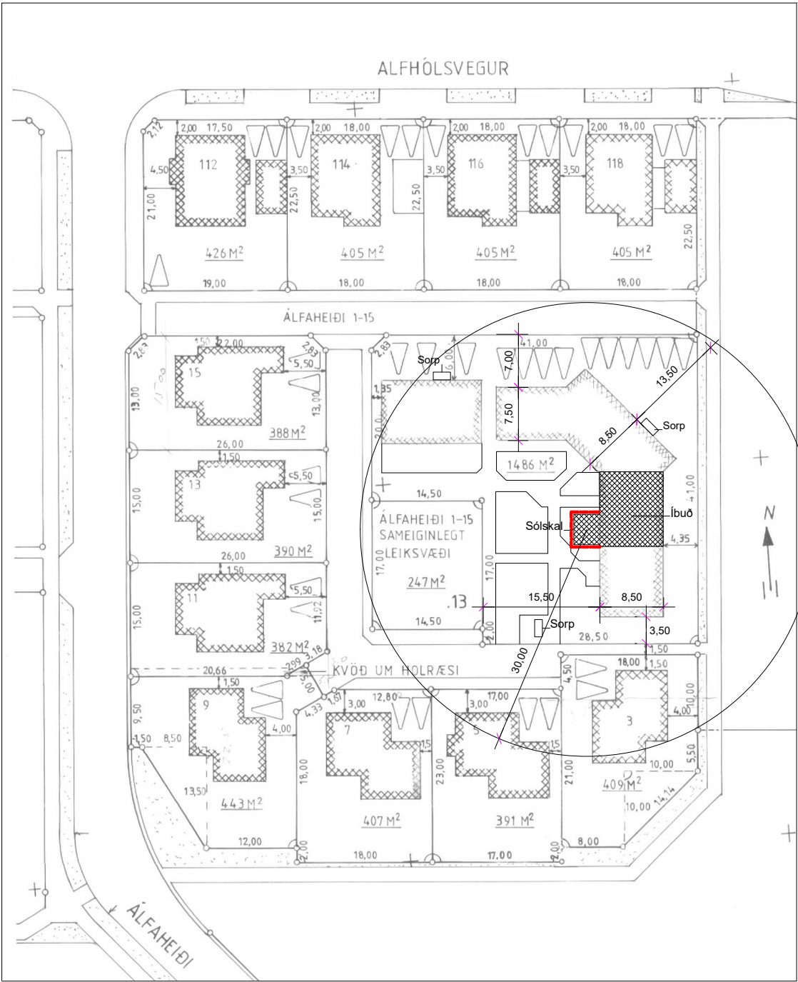
Afstöðumynd - Mkv. 1:500
