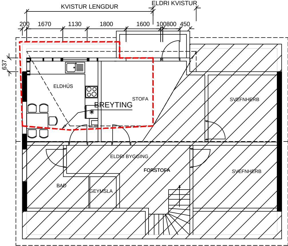
GRUNNMYND ÞAKHÆÐ, mkv.1:100
