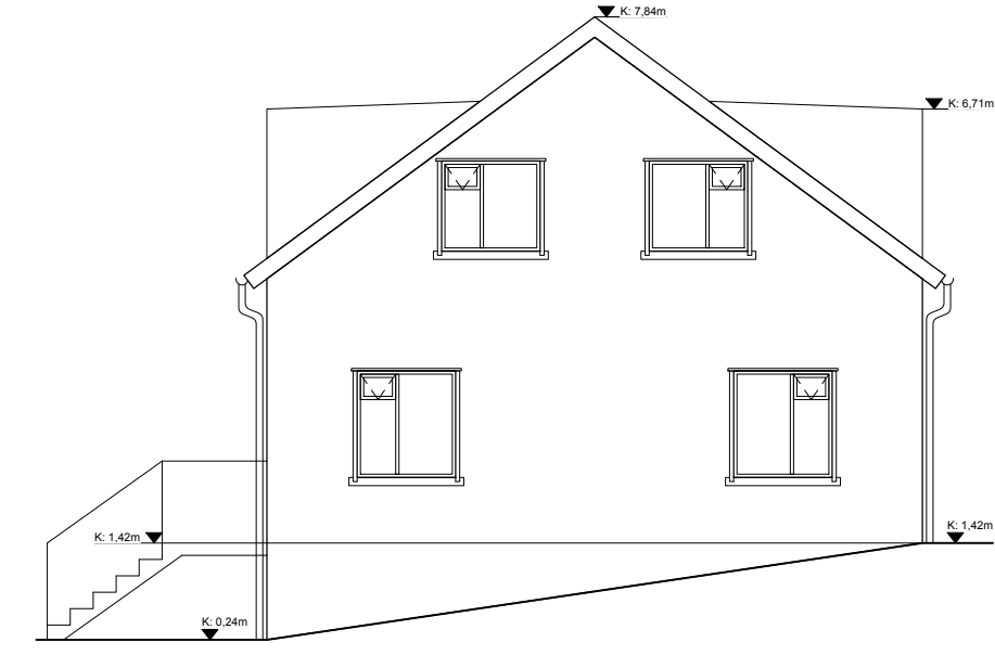
VESTURHLÍÐ 1:100
