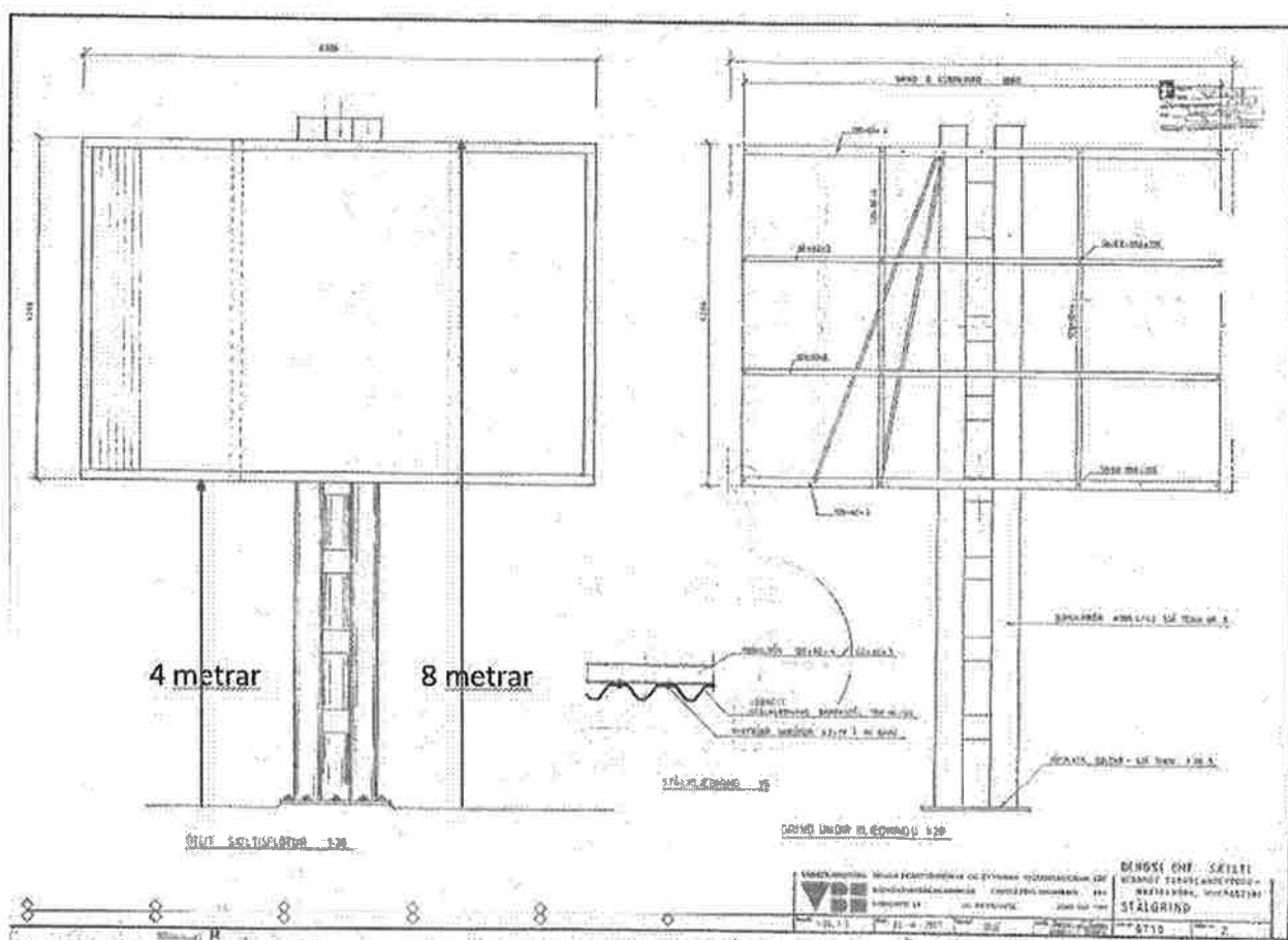
Figure 1 Teikning af skilti og burðarvirki
