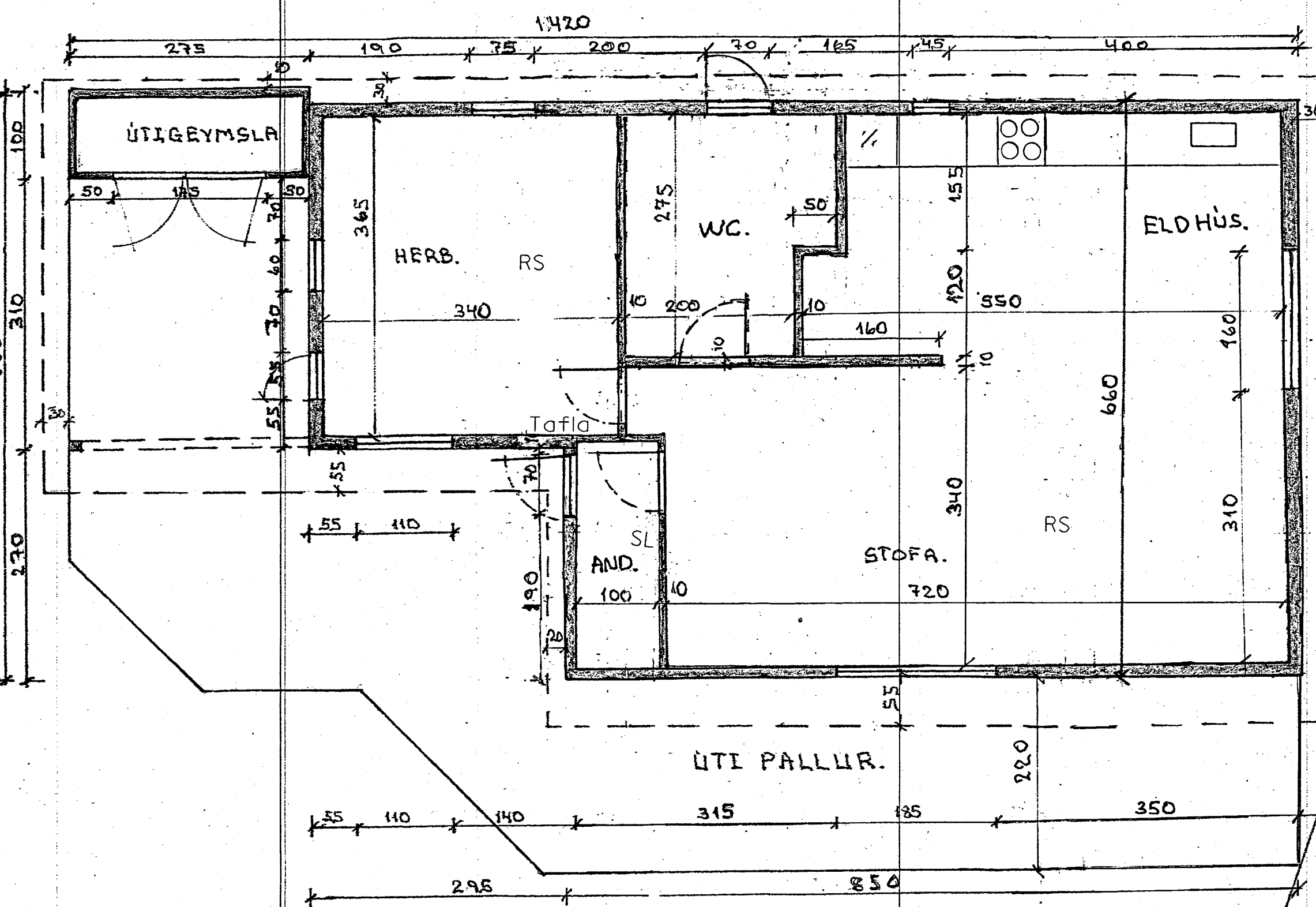
GRUNNMYND.
