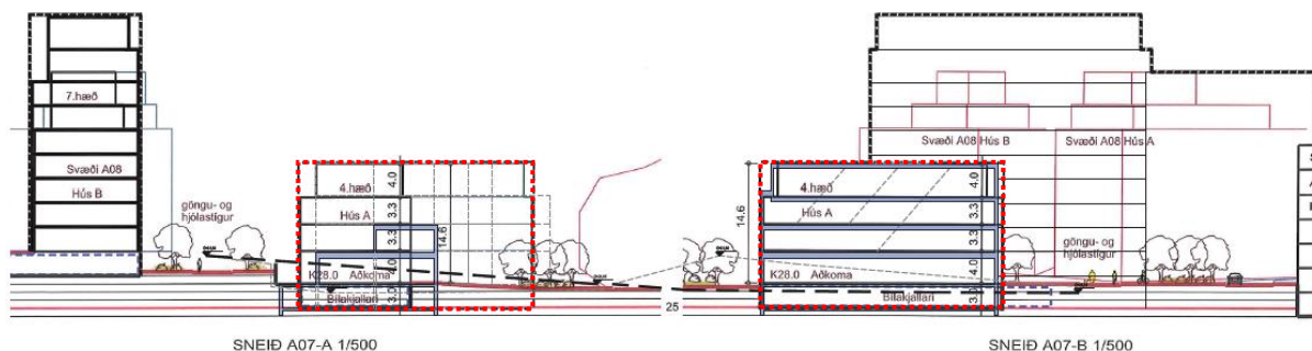
Mynd 3. Sneiðingar úr gildandi deiliskipulagi. Rauðar strikálínur sýna hámarksbyggingarreit, bláa formið sýnir mögulegar útlínur og hæðir á forhönnun Batterísins á Silfursmára 12 og rauðu punktalínurnar ytri mörk gildandi byggingarreits.
