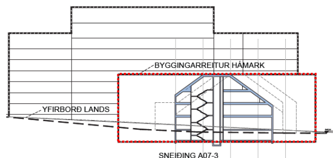
Mynd 4. Nýtt snið vegna forhönnunar. Sniðið sýnir í bakgrunni Sunnasmára 13 og 11. Útlínur byggingarreits skv gildandi deiliskipulagi er sýndur með rauðri strikálínu (Byggingarreitur hámark). Innan byggingarreits S12 má sjá mögulegar útlínur og hæðir forhönnunar fyrir Silfursmára 12 (blátt form og strikpunktalínur).
