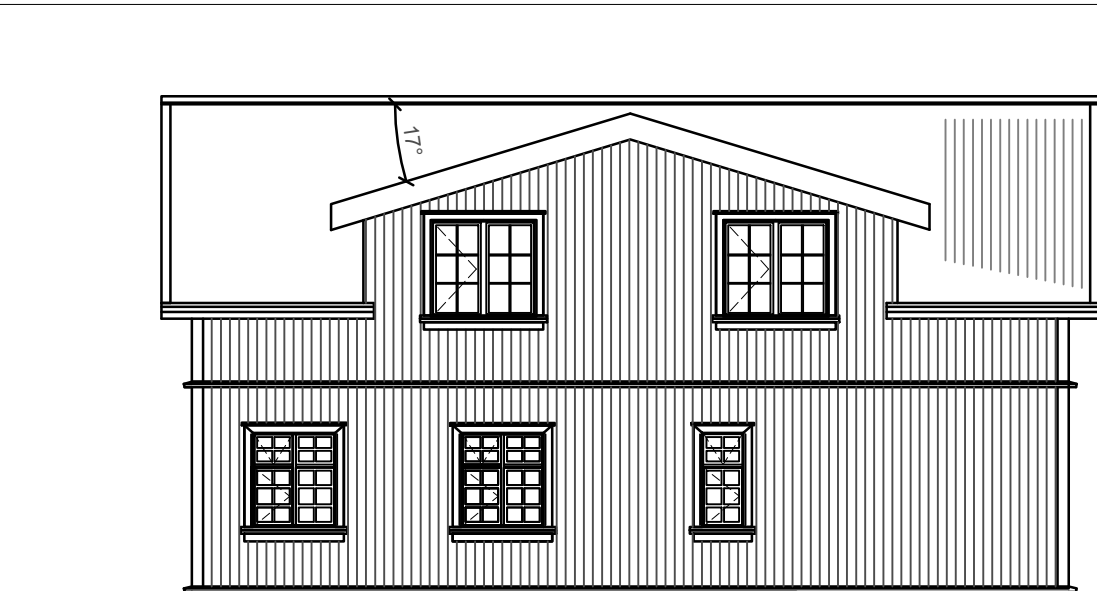
Útlit Norður
