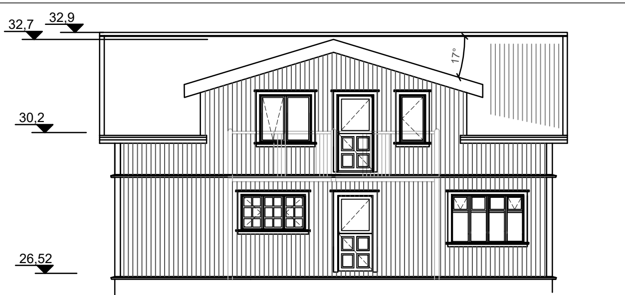
Útlit Suður
