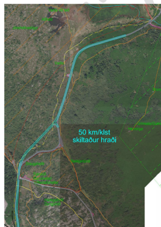
MYND 12 Fyrstu drög að legu Elliðavatsnsvegur við Stekkjartún þar sem leyfilegur hámarkshraði er 50 km/klst. Lega vegar yrði útfærð nánar á síðari stikum.
