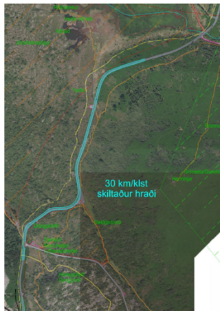
MYND 11 Fyrsta tillaga að legu Elliðavatsnsvegur við Stekkjartún/Mariuhella með leyfilegum hámarkshraða 30 km/klst.
