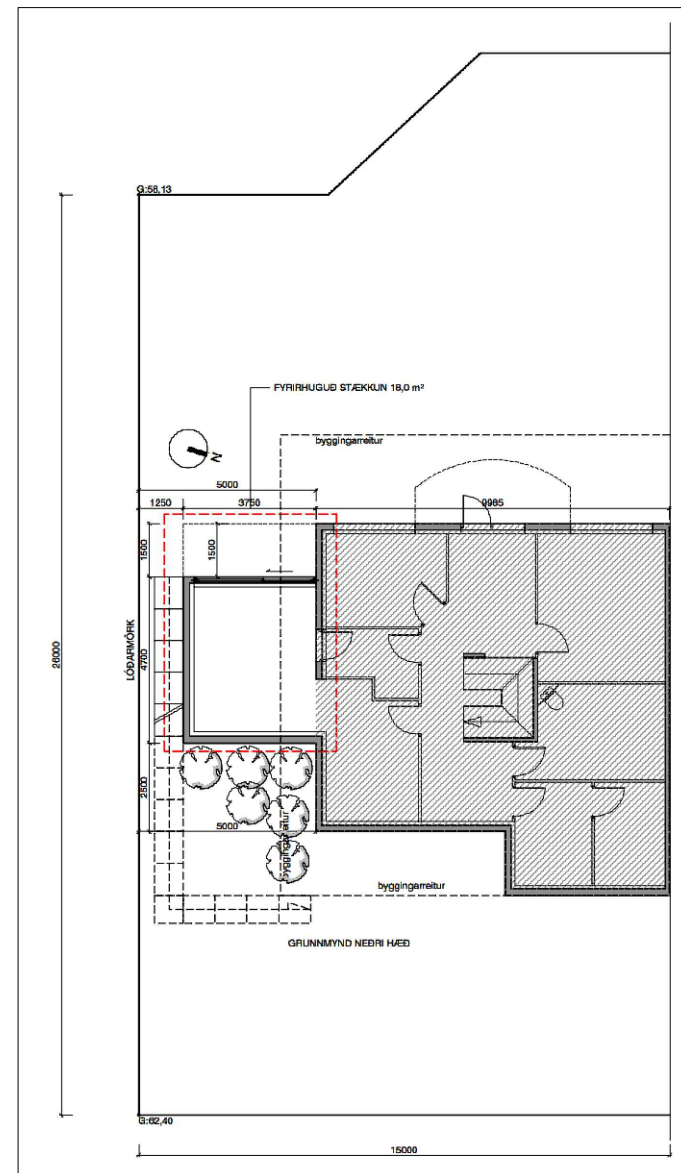
Skýringarmynd: Tillaga - Grunnmynd neðri hæðar mkv. 1:200
