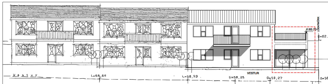
Skýringarmynd: Tillaga - Útlit til vesturs.
