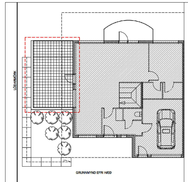
Skýringarmynd: Tillaga - Grunnmynd efri hæðar mkv.1:200
