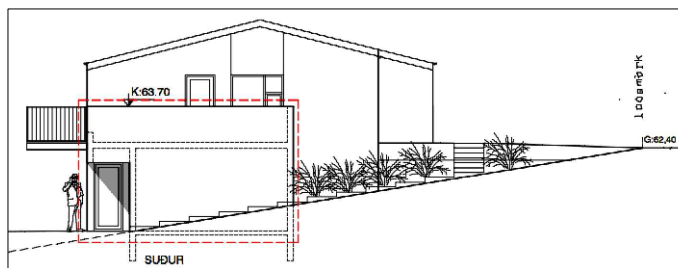
Skýringarmynd: Tillaga - Útlit til suðurs.
