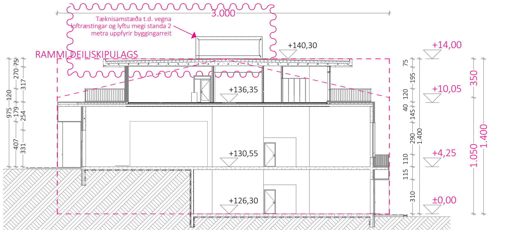
SKILMÁLAR SNÍÐ A 1:200
