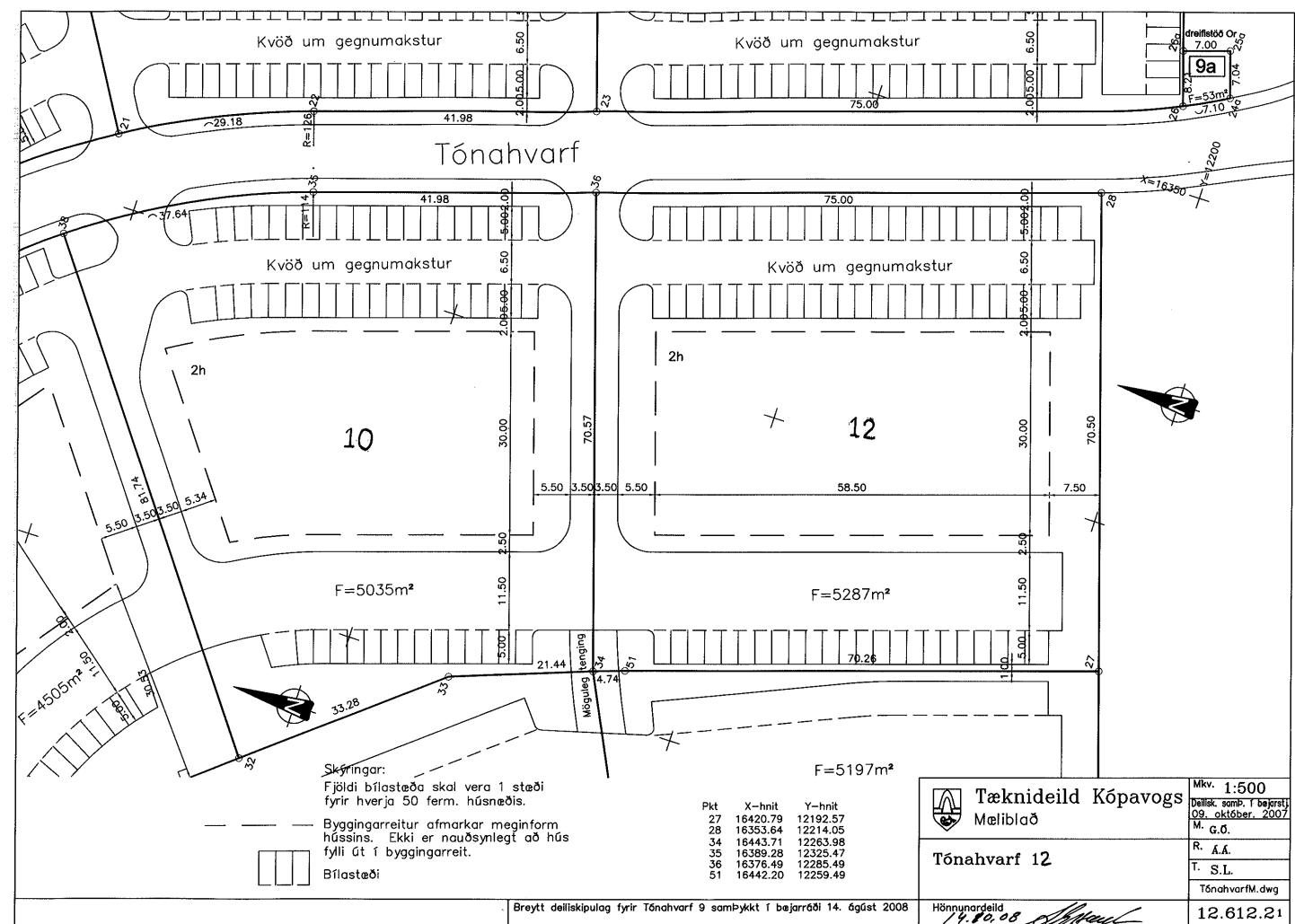
Tónahvarf 12 Mælibleið 1 (2078) 1:2
