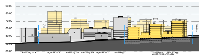
SKILMÁLARSNEIÐING C-C DIGRANESVEGUR
