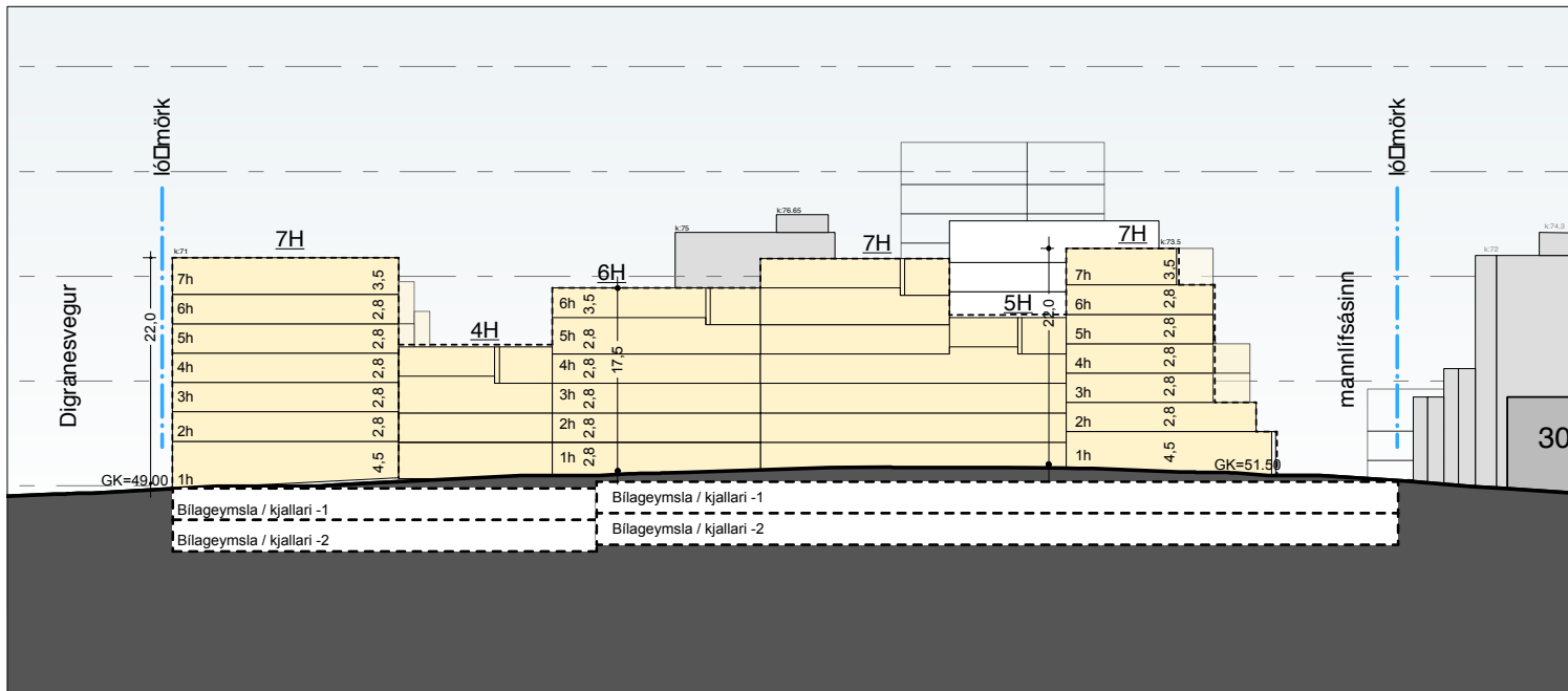
SNÍÐ A-A, mkv 1:500 (A3)
