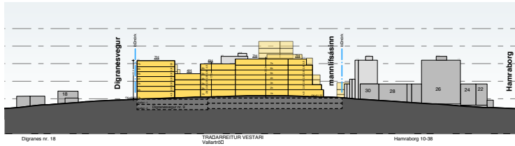
SKILMÁLARSNEIÐING A-A VALLARTRÖÐ
