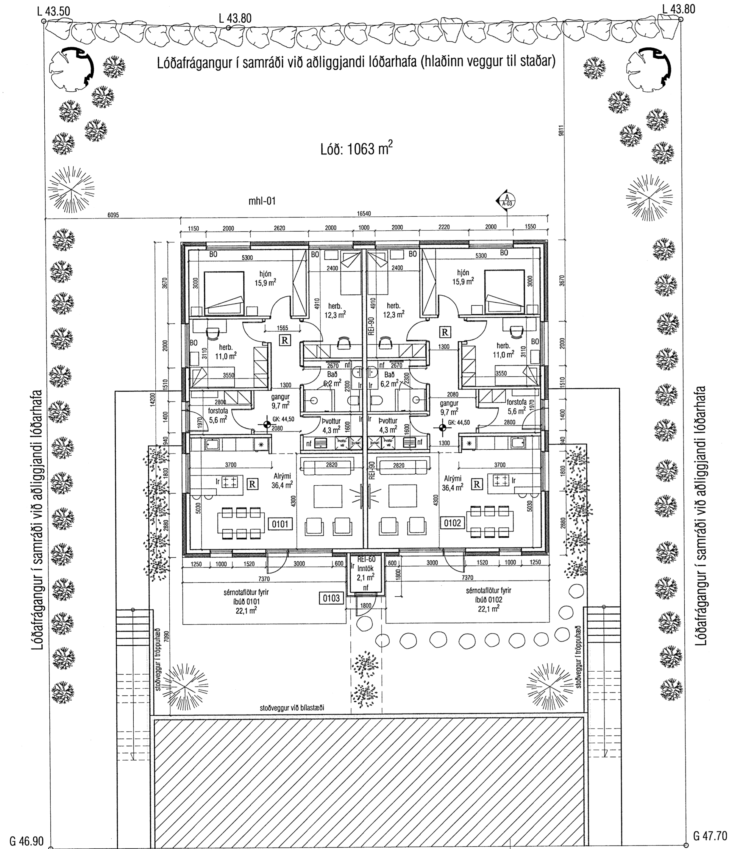
Grunnmynd 1.hæð
