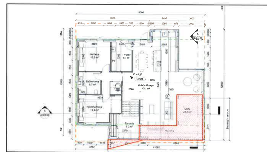
Tillaga að breyttu deiliskipulagi: Grunnmynd efri hæð í mkv. 1:250
