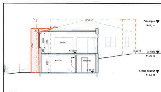
Skýringarmynd: Útlit snið a:a í mkv. 1:250
