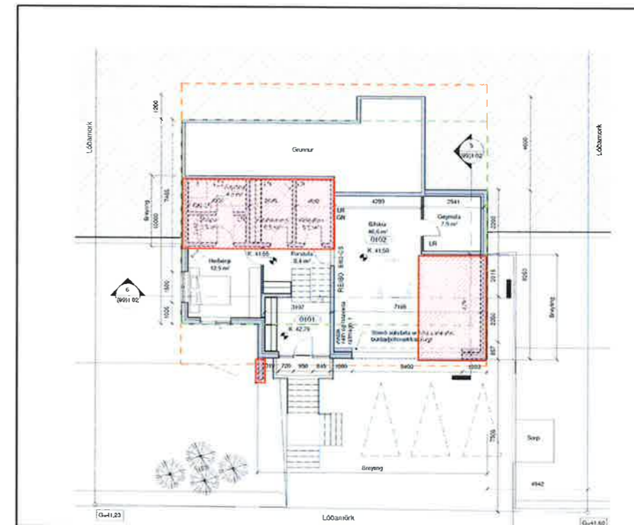
Tillaga að breyttu deiliskipulagi: Grunnmynd neðri hæð í mkv. 1:250
