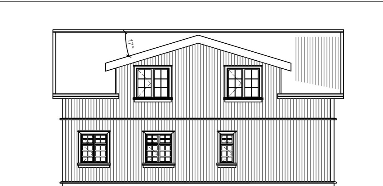
Útlit Norður
