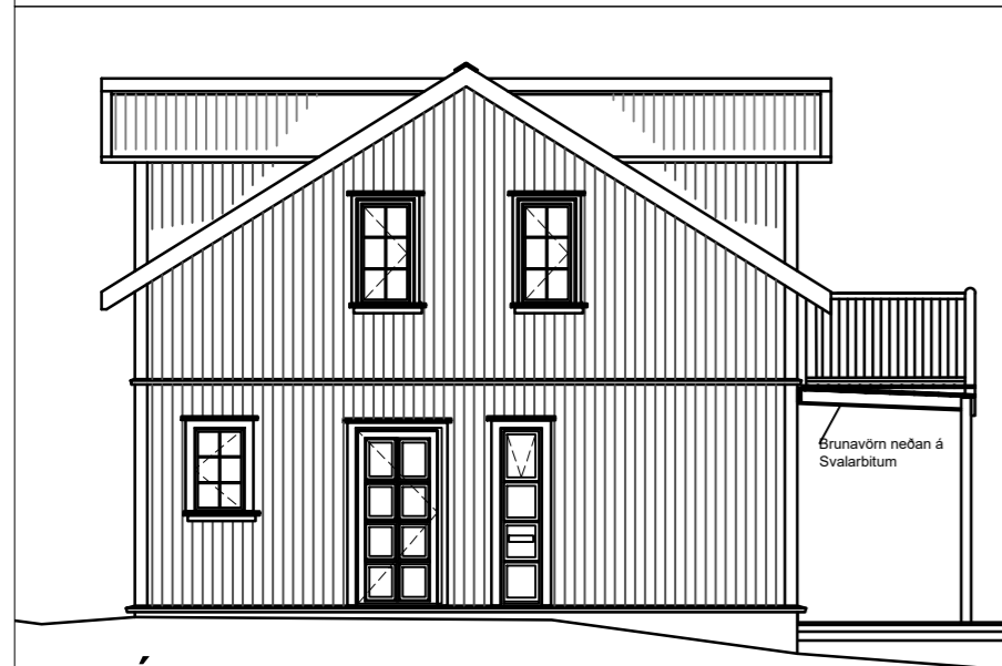
Útlit Vestur
