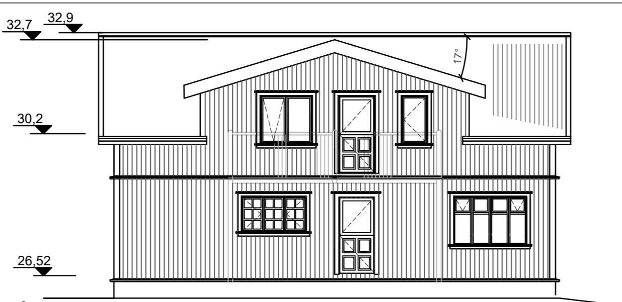
Útlit Suður
