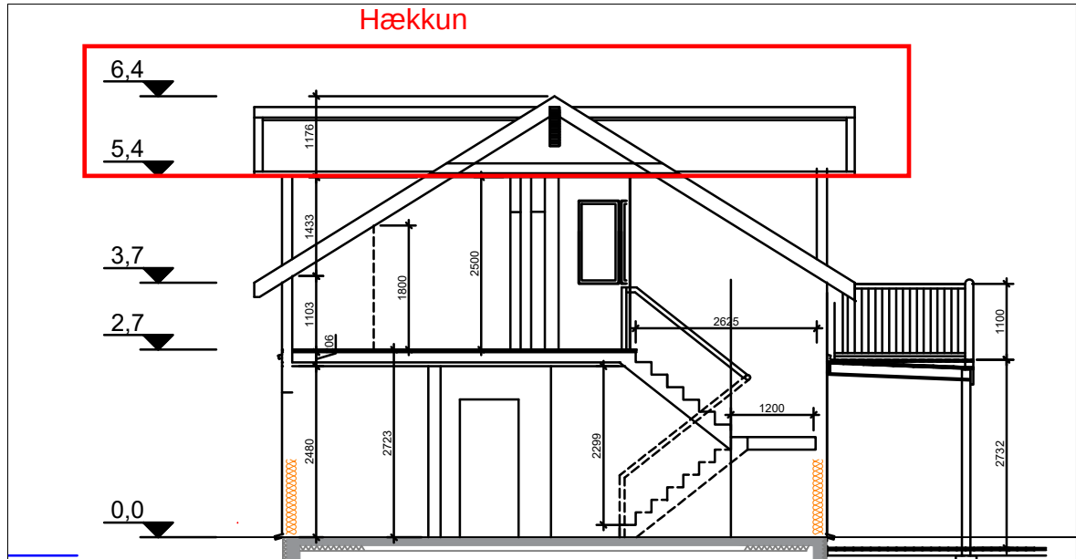
Snið A-A
