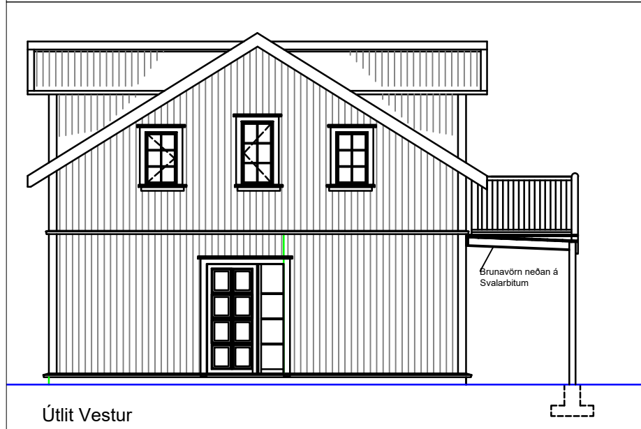
Útlit Vestur
