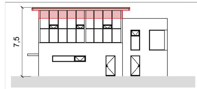
Skýringarmynd: Suðvestur útlit í mkv. 1:250
