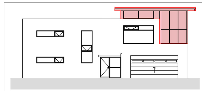
Skýringarmynd: Norðvestur útlit í mkv. 1:250
