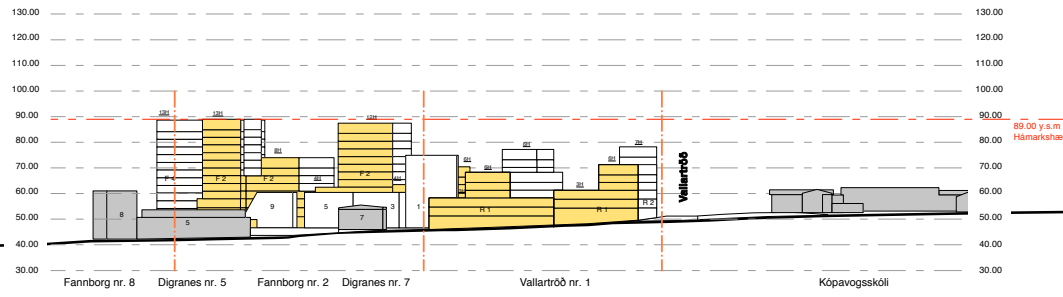
SKILMÁLARSNEIÐING C-C DIGRANESVEGUR
